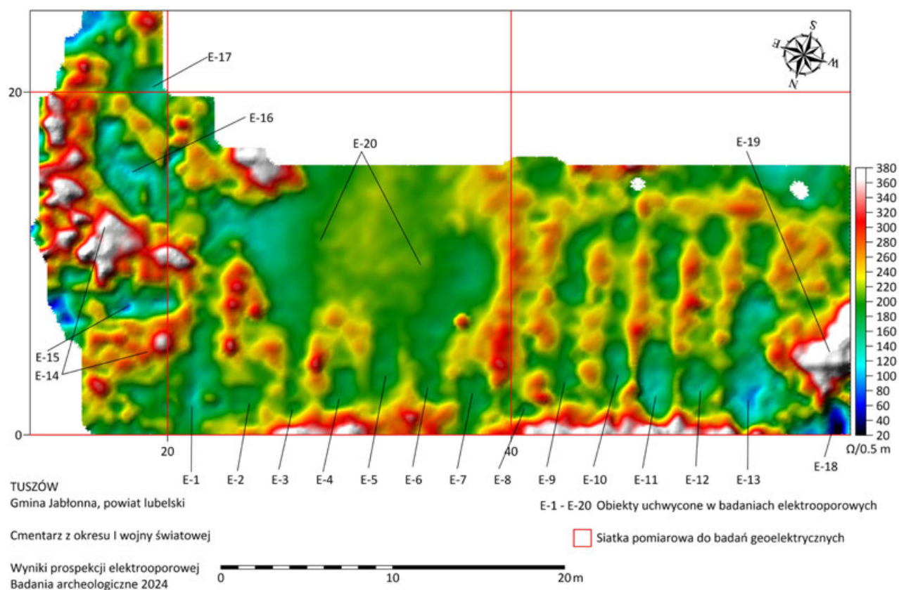
Ryc. 7. Tuszów, gmina Jabłonna, powiat lubelski. Cmentarz z okresu pierwszej wojny światowej. Wyniki prospekcji elektrooporowej z oznaczeniem zidentyfikowanych obiektów archeologicznych. Oprac. M. Piotrowski
