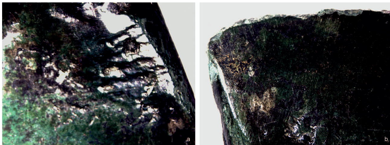
Ryc. 5. Siekierka z Falejówki, obraz makroskopowy ostrza: a – ślady obróbki powierzchniowej na zewnętrznej ścianie tulei w pobliżu płaszczyzny ostrza; b – część tnąca i zakończenie ostrza ze śladami szlifowania powierzchni. Oprac. A. Garbacz-Klempka, P. Jurecki Fig. 5. Falejówka axe, macroscopic image of the blade: a – traces of surface treatment on the outer wall of the socket near the plane of the blade; b – cutting part and tip of the blade with traces of surface grinding. Developed by A. Garbacz-Klempka, P. Jurecki
