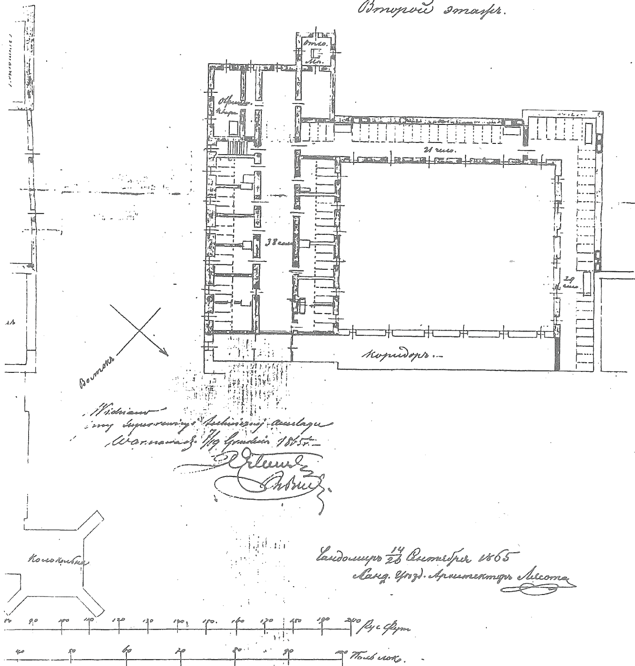
Рис. 12. Plan klasztoru podominikańskiego wg pomiaru arch. J. Lasoty z 1865 roku, rzut piętra, oryg. AP Radom RGR 4265 ABB. 12. Plan des Postdominikanerklosters nach architektonischer Messung von Jan Lasota aus dem Jahre 1865, Grundriß des Stockwerks, Original Staatsarchiv Radom RGR 4265
