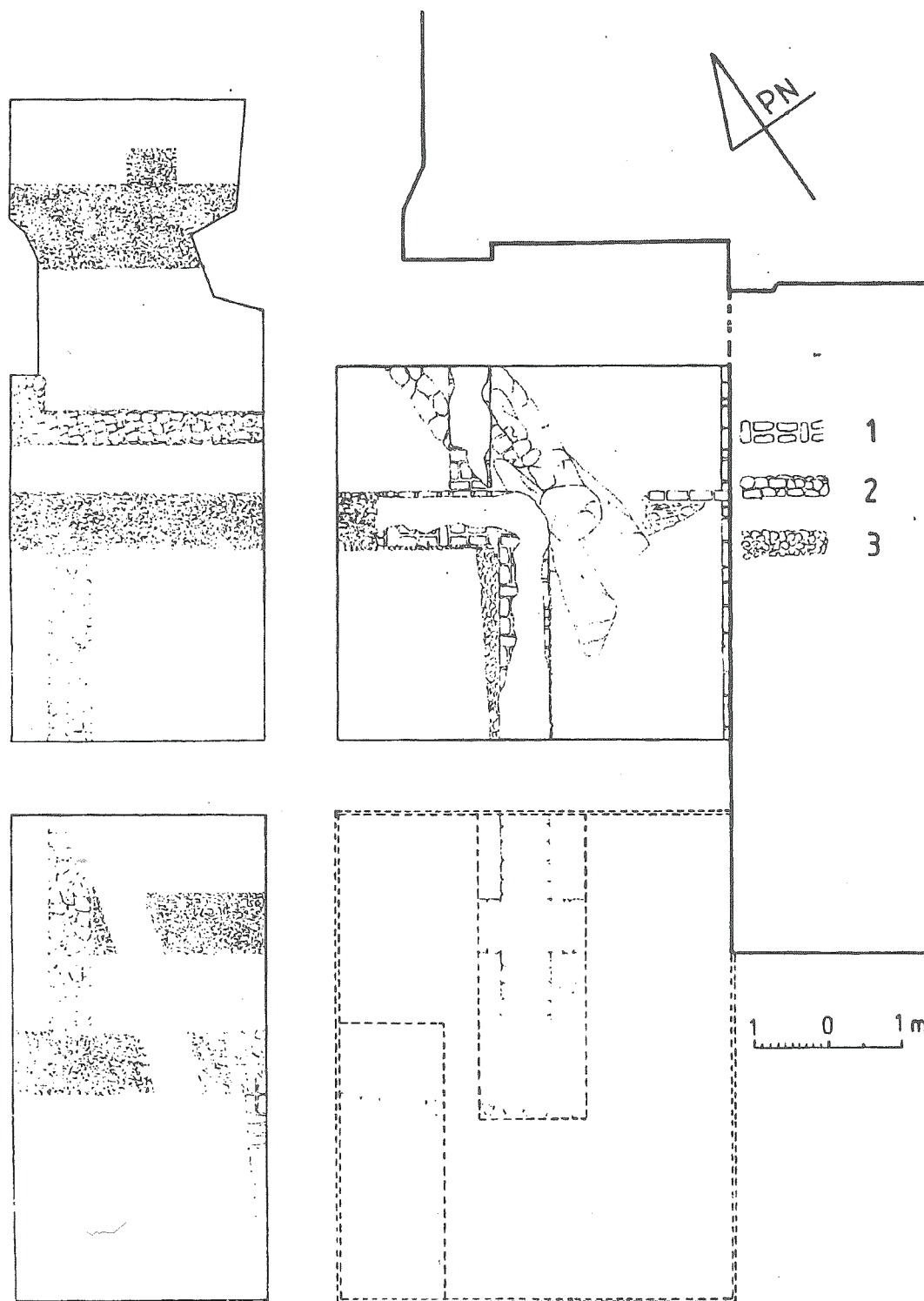
Ryc. 16. Plan odsłoniętych murów i fundamentów, także czytelnych w negatywach; oznaczenia: 1 — mur ceglany, 2 — mur kamienny, 3 — negatyw muru (fundamentu)
