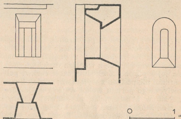
Ryc. 5. Posada Rybotycka pow. Przemyśl. Cerkiew, strzelnica nad nawą.
