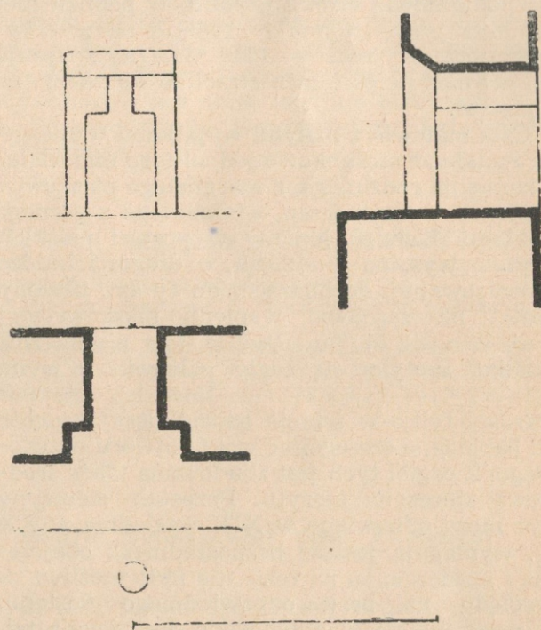
Ryc. 6. Posada Rybotycka pow. Przemyśl, Cerkiew, strzelnica w szczycie.
