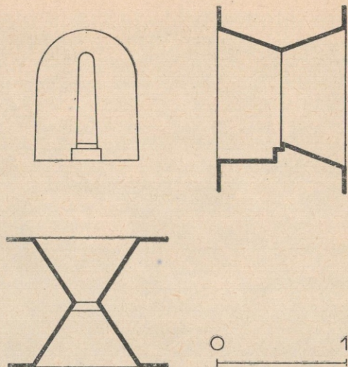
Ryc. 4. Posada Rybotycka pow. Przemyśl. Cerkiew, strzelnica na I piętrze wieży.
