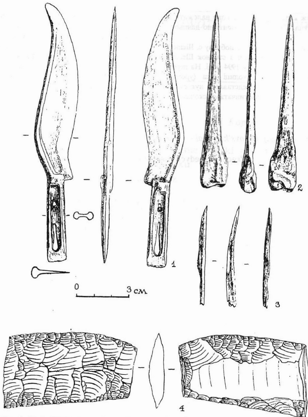
Рис. 2. Одаїв XVIII. Епоха бронзи (= т.з. тракійський гальштат):
