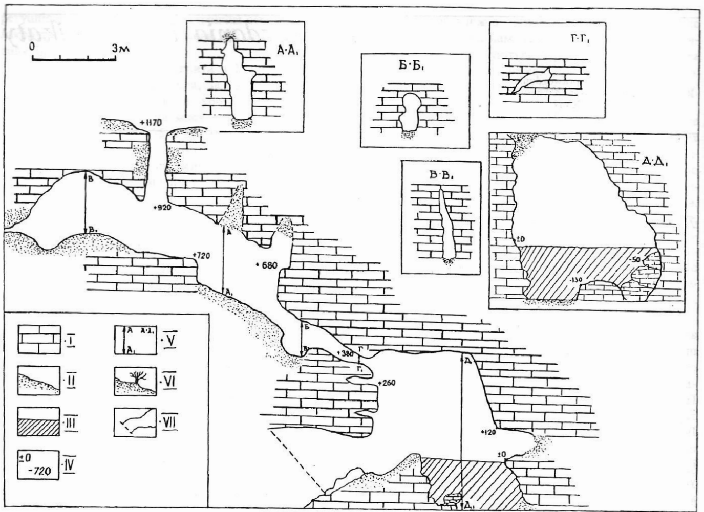
Рис. 1. Комплекс Одаїв XVII (Печера Затишна — А. Битиновича):
