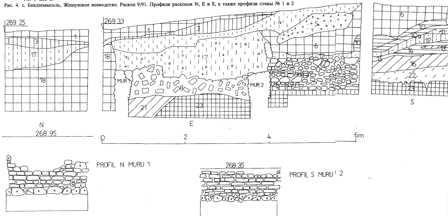
Ryc. 4. Będziemyśl, woj. Rzeszów, stan. 1. Wykop 9/91. Profile wykopu N, E i S oraz profile muru nr 1 i 2 Abb. 4. Będziemyśl, Wojewodschaft Rzeszów, Fundstelle 1. Ausgrabung 9/91. Ausgrabungsprofile N, E und S sowie Mauerprofile Nr. 1 und 2.
