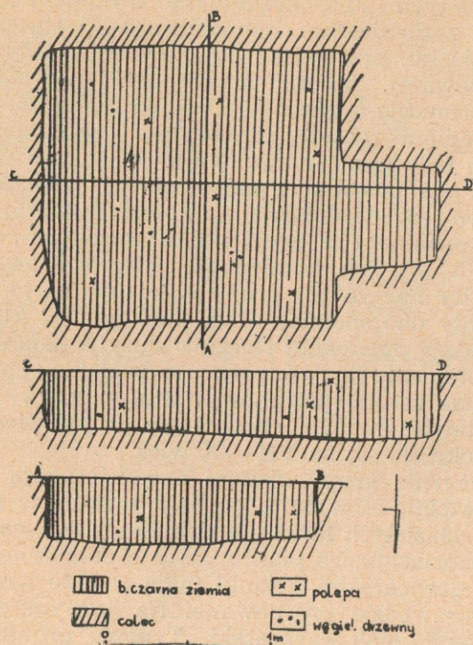
Ryc. 1. Rzeszów — Staromieście, stan. nr 3. Rzut poziomy i profile jamy nr 36.
