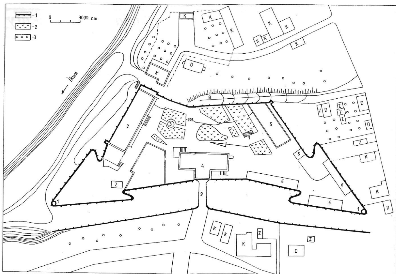
Ryc. 1. Plan zamku w Dubnie
