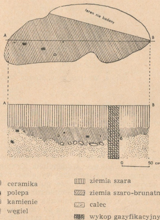
Ryc. 6. Wietrznie pow. Krosno. Wykop W II/1966 r. Plan i profil jamy J III/1966 r.
