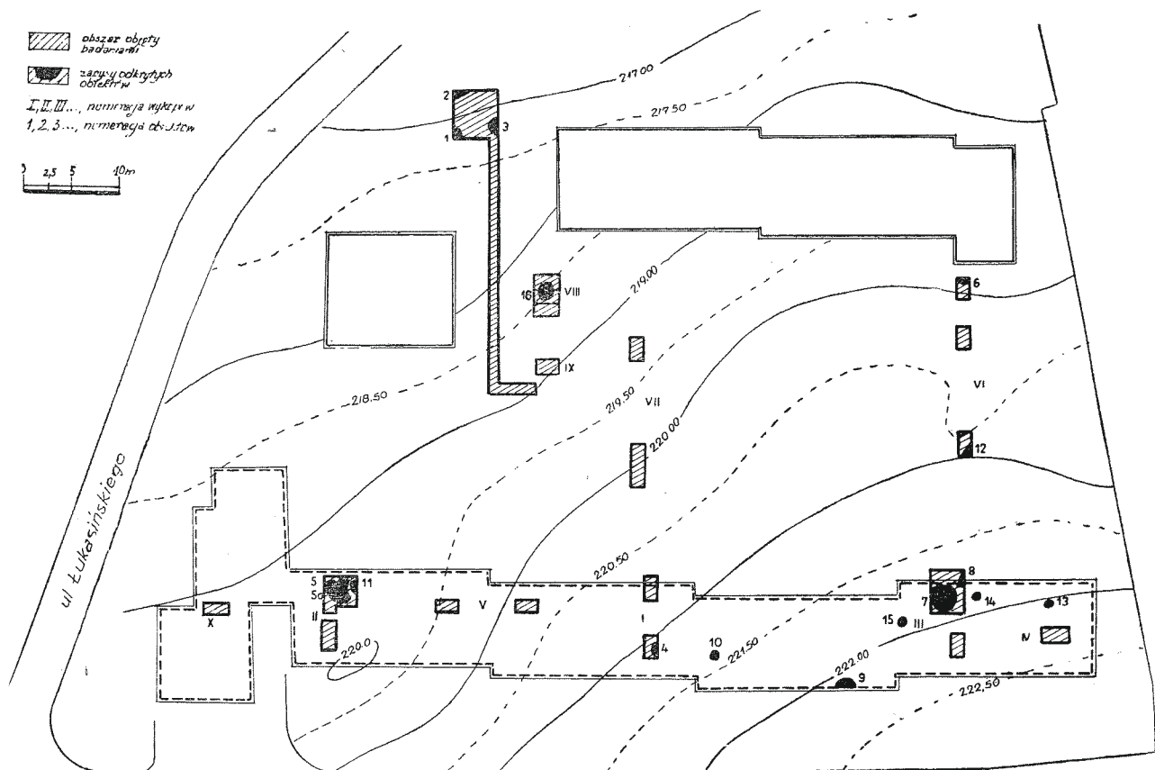
Ryc. 1. Przemyśl, ul. Łukasińskiego. Plan sytuacyjno-wysokościowy wykopów i odkrytych obiektów archeologicznych.
