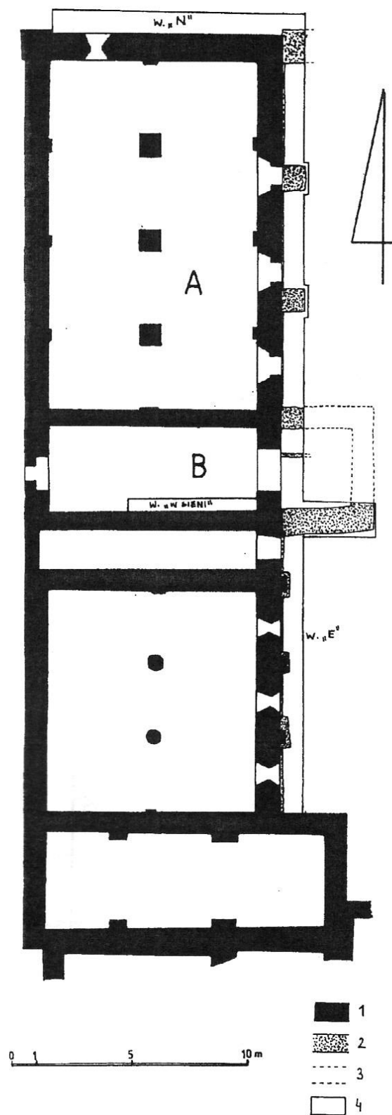
Рис. 3. Копrzywnica — zespół pocysterski, dawny budynek klasztoru — plan wykopów oznaczenia: A — Frateria, B — Sien przelotowa, 1 — mury parteru, 2 — mury odsłonięte w wykopach, 3 — mury o przebiegu rekonstruowanym, 4 — granice wykopów
