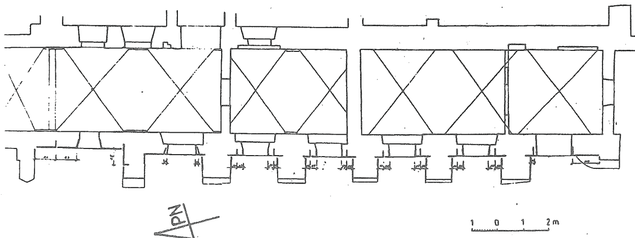
Ryc. 2. Rzut parteru zachodniej części wschodniego skrzydła klasztornego — inwentaryzacja wyników badań Abb. 2. Grundriß vom Erdgeschoß westlicher Seite des östlichen Klosterflügels — Inventur der Forschungsergebnisse Рис. 2. Проекция партера западной части восточного монастырского крыла — инвентаризация итогов исследований
