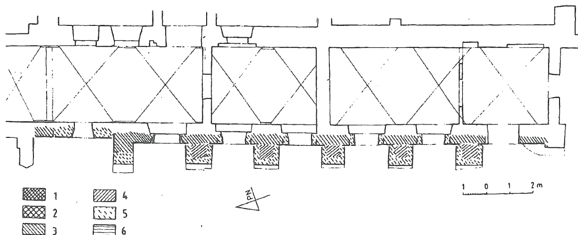
Ryc. 5. Rzut parteru zachodniej części wschodniego skrzydła klasztornego — interpretacja wyników badań; oznaczenia: 1—2 poł. XIII wieku, 2—2 poł. XIV wieku, 3—3/4 ćw. XVII wieku, 4—2 ćw. XVIII wieku (ok. 1734 roku), 5 — po 1864 roku, 6 — po 1905 roku
