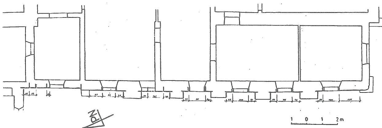
Ryc. 3. Rzut piętra zachodniej części wschodniego skrzydła klasztornego — inwentaryzacja wyników badań Abb. 3. Grundriß des Stockwerks westlicher Seite des östlichen Klosterflügels — Inventur der Forschungsergebnisse Рис. 3. Проекция этажа западной части восточного монастырского крыла — инвентаризация итогов исследований
