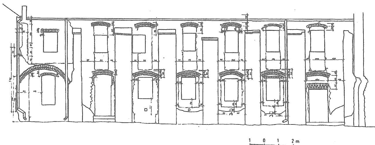
Ryc. 4. Elewacja zachodnia wschodniego skrzydła zabudowań klasztornych — inwentaryzacja wyników badań Abb. 4. Westliche Fassade des östlichen Flügels der Klostergebäuden — Inventur der Forschungsergebnisse Рис. 4. Западный фасад восточного крыла монастырских застроек — инвентаризация итогов исследований
