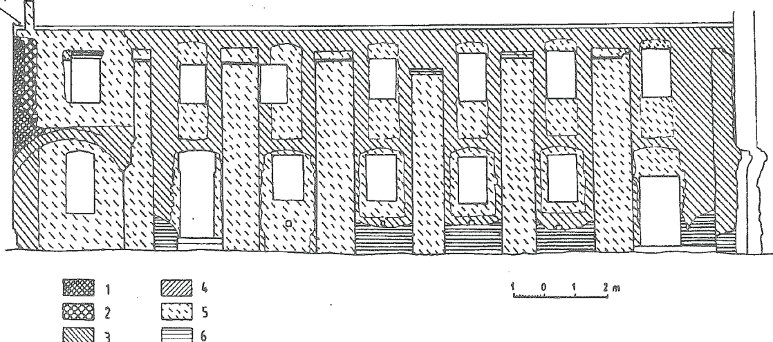
Ryc. 7. Elewacja zachodnia wschodniego skrzydła zabudowań klasztornych — interpretacja wyników badań; oznaczenia jak w ryc. 5
