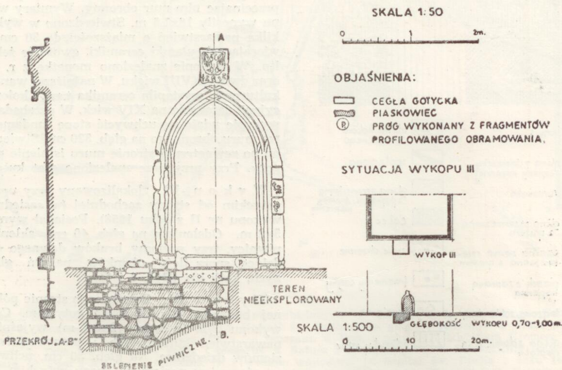
Ryc. 4a. Biecz pow. Gorlice. Profil gotyckiego portalu oraz wykopu nr III przy Szpitalu św. Ducha.
