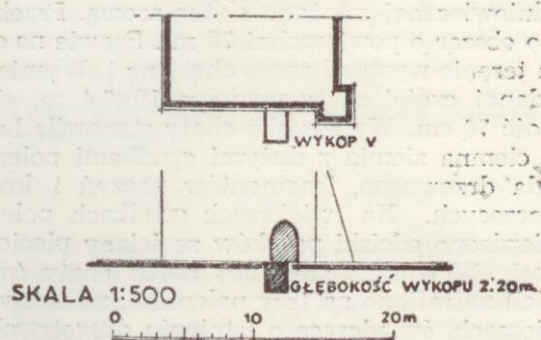
Ryc. 5. Biecz pow. Gorlice. a) Portal gotycki w północnej ścianie Szpitala św. Ducha oraz południowy profil wykopu nr IV. b) Czwór gotycki w ścianie wschodniej Szpitala św. Ducha oraz wschodni profil wykopu nr V.
