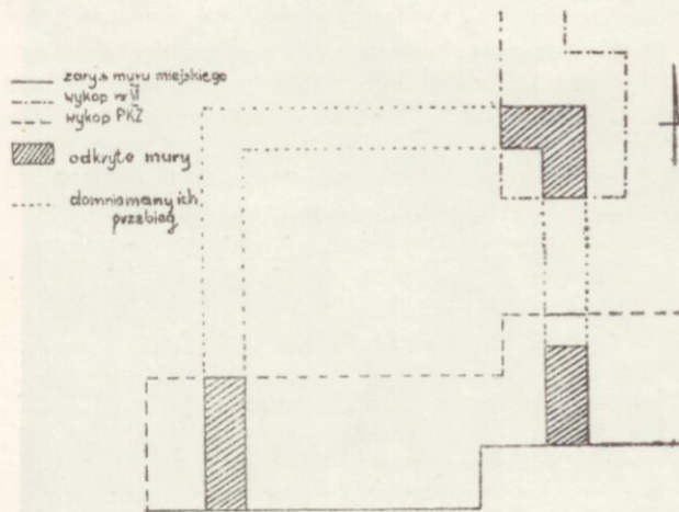
Ryc. 3. Biecz pow. Gorlice. Rzut poziomy odkrytych murów zagadkowej budowli, domniemany jej zarys. Skala 1:200.
