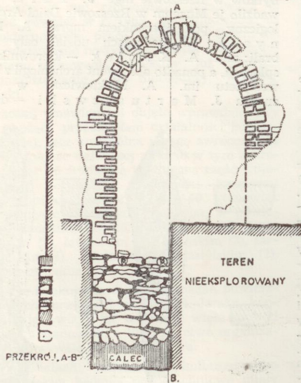
Ryc. 5. Biecz pow. Gorlice. a) Portal gotycki w północnej ścianie Szpitala św. Ducha oraz południowy profil wykopu nr IV. b) Czwór gotycki w ścianie wschodniej Szpitala św. Ducha oraz wschodni profil wykopu nr V.
