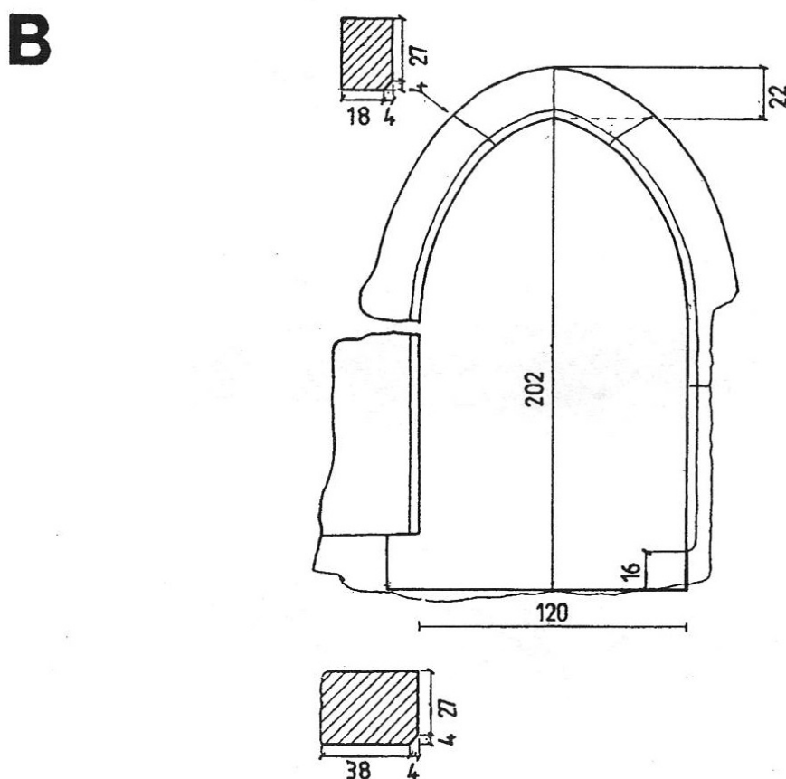
Ryc. 2. Czchów – zamek, A – lico ściany północnej klatki schodowej z portalem gotyckim – wejściem do piwnic zamkowych, B – kamienny portal gotycki (rys. A. Michta)
