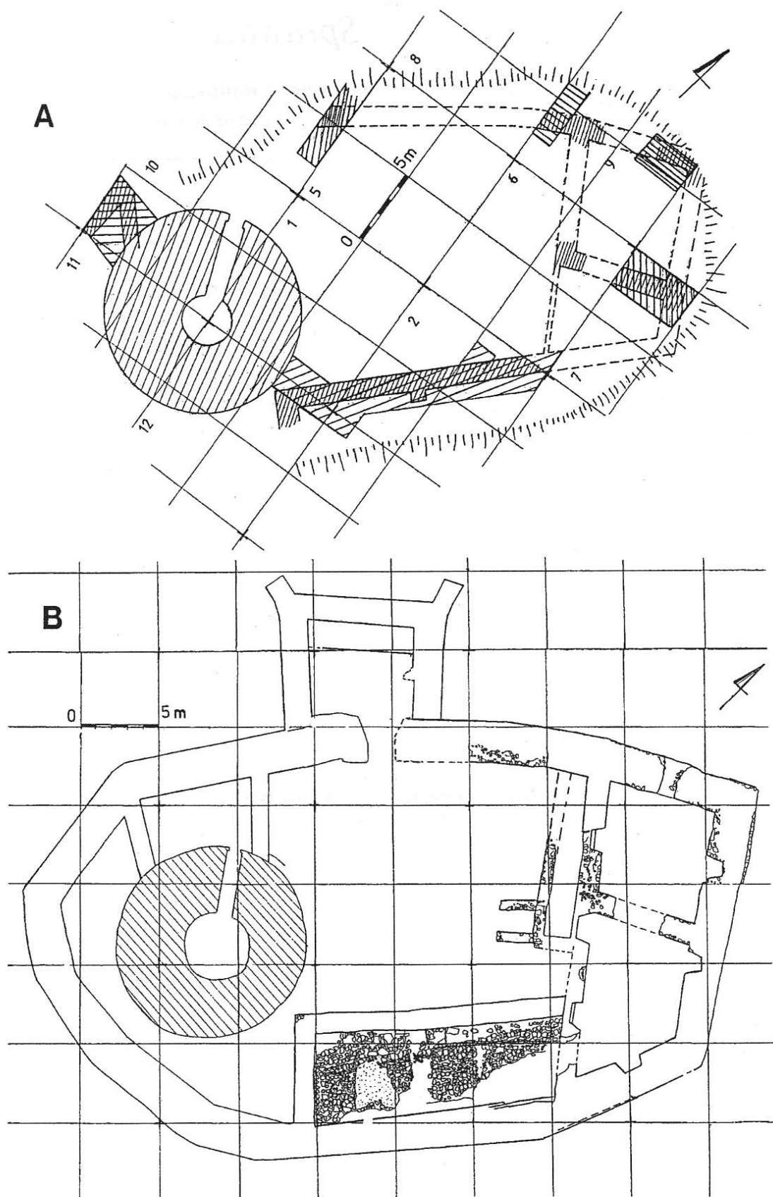
Ryc. 1 Czchów – zamek, A – plan zabudowy wzgórza zamkowego wg. A. Żakiego z naniesionymi sondami i siatką arową. B – zamek, plan zabudowy wzgórza zamkowego w Czchowie po badaniach w latach 1993–1999 (rys. A. Michta)
