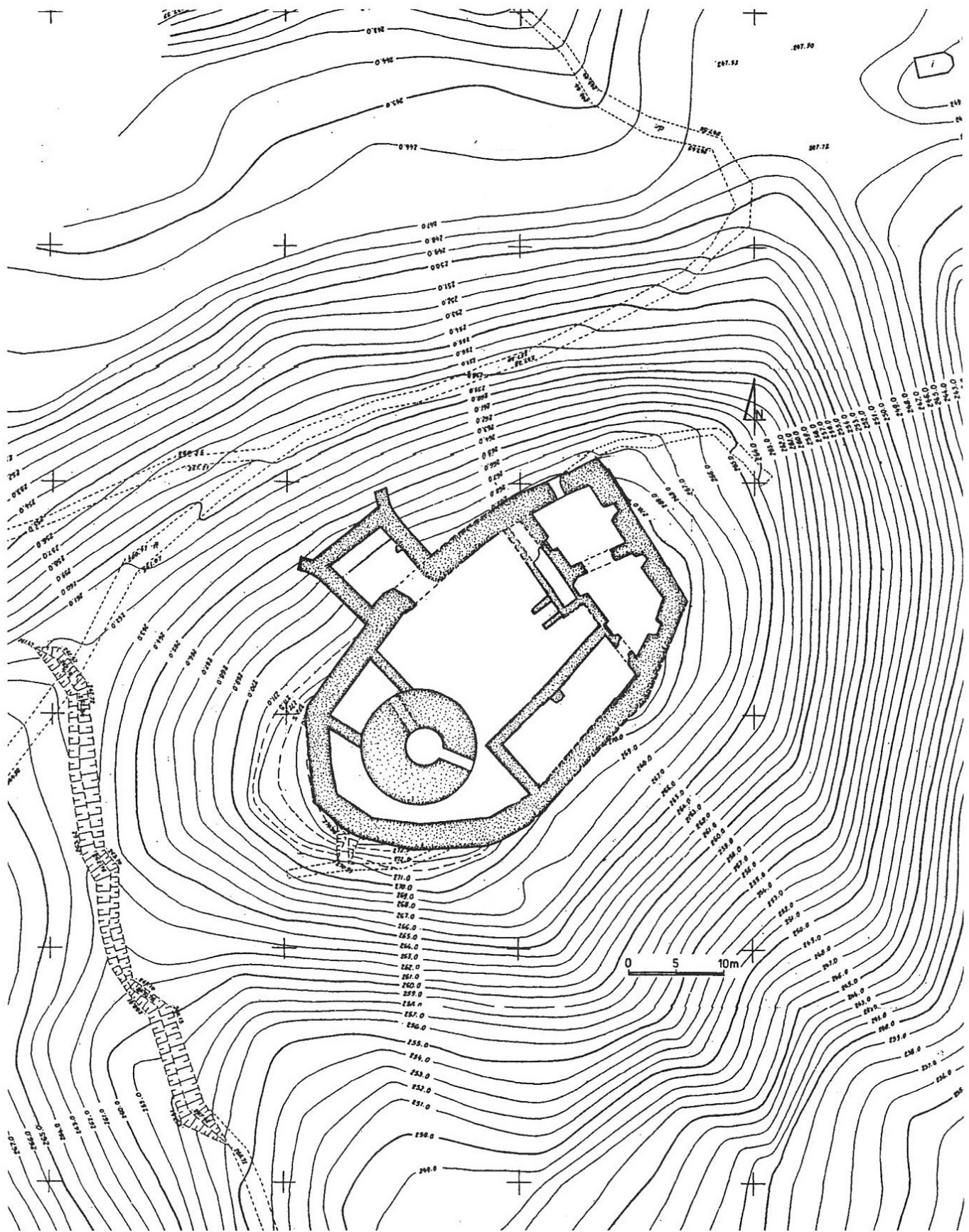
Ryc. 4. Czchów – zamek, zabudowa wzgórza zamkowego na planie warstwicowym. (rys. A. Michta)
