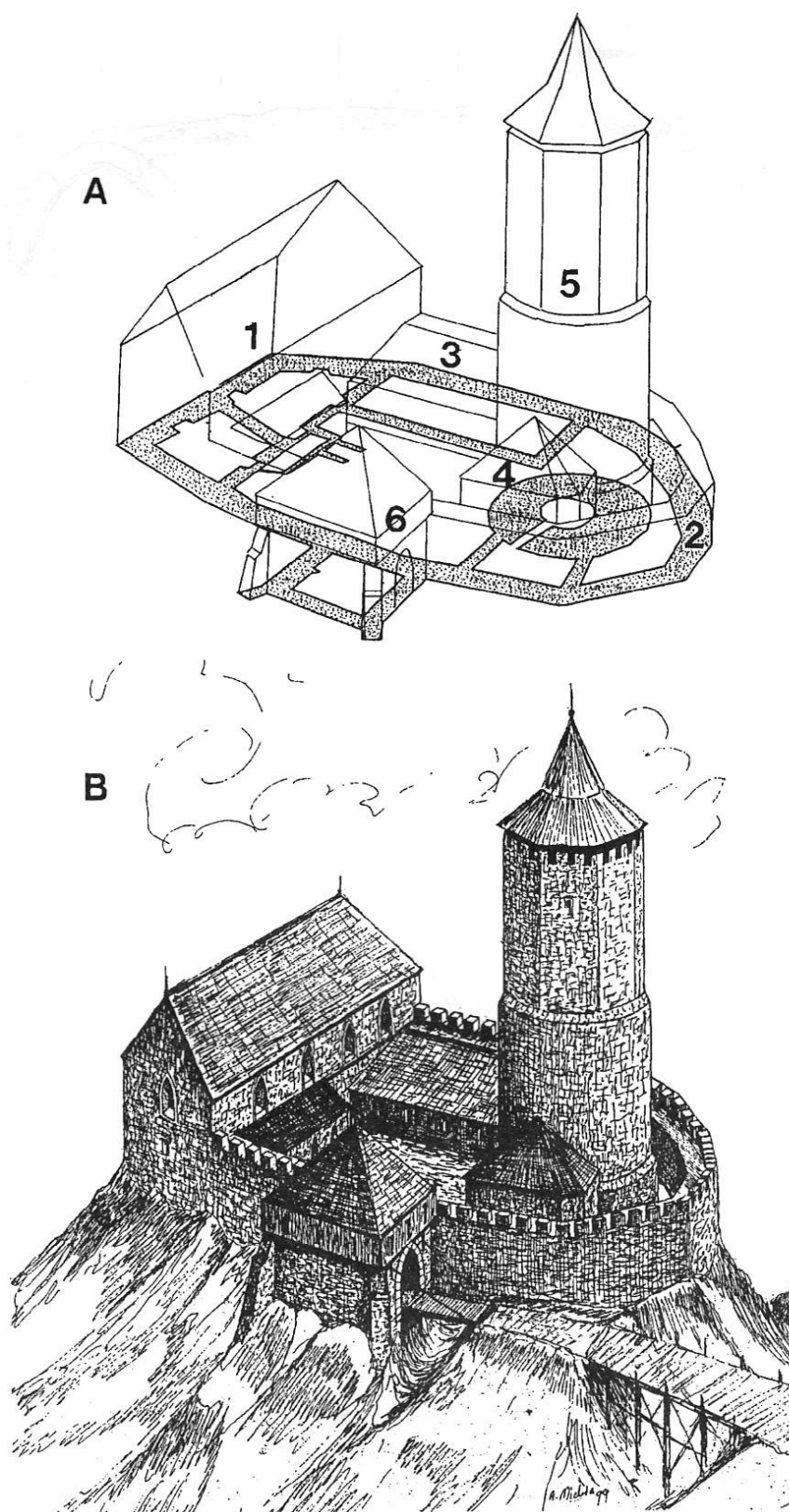
Ryc. 3. Czchów – zamek, A – bryły głównych elementów budowli naniesione na przetworzony plan fundamentów (1 – dom zamkowy, 2 – mury obwodowe, 3 – budynek zachodni, 4 – budynek przy wieży, 5 – wieża, 6 – budynek bramy), B – artystyczna rekonstrukcja zamku wg A. Michty
