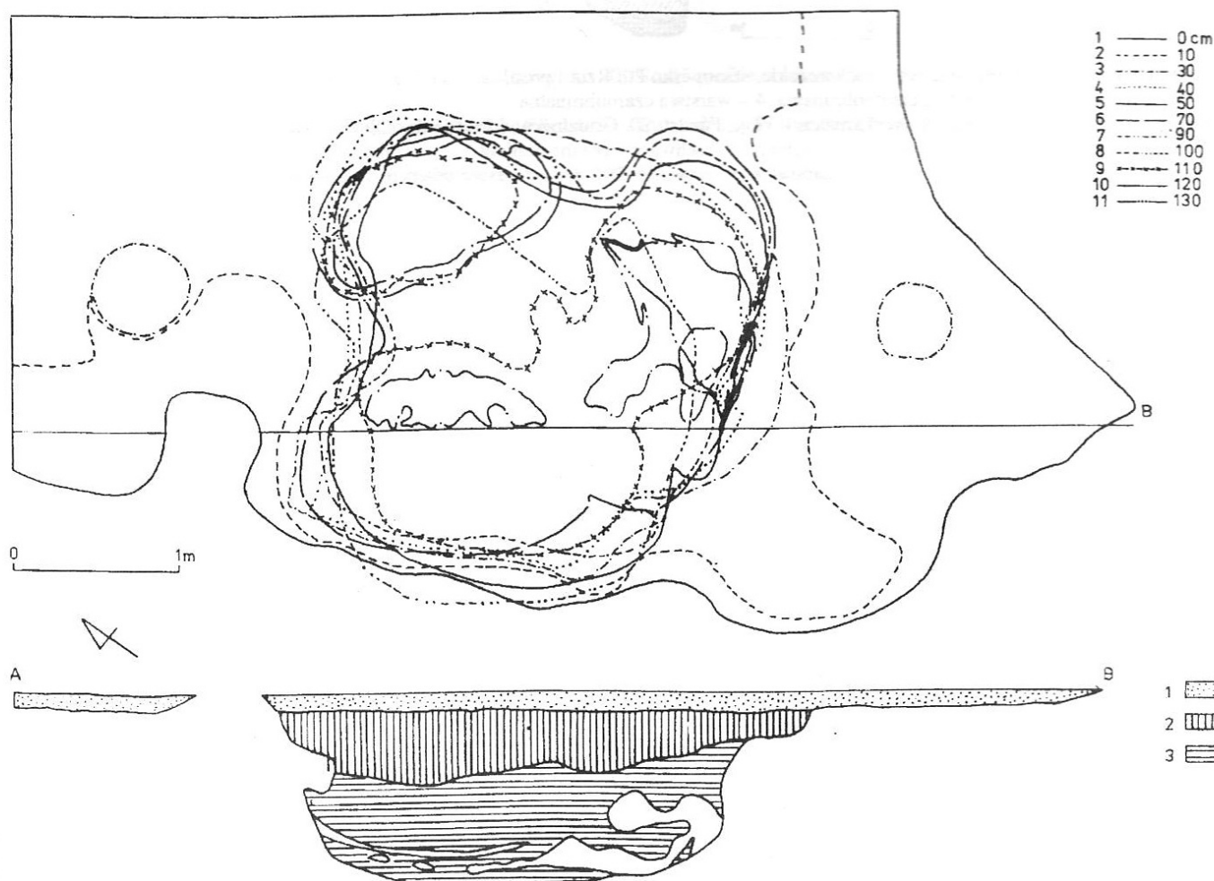
Rys. 8. Olchowa, gm. Iwierzycze, woj. podkarpackie, stanowisko 20. Rzut i profil obiektu 2; 1 – warstwa beżowa, 2 – warstwa jasnobrunatna, 3 – warstwa ciemnobrunatna
