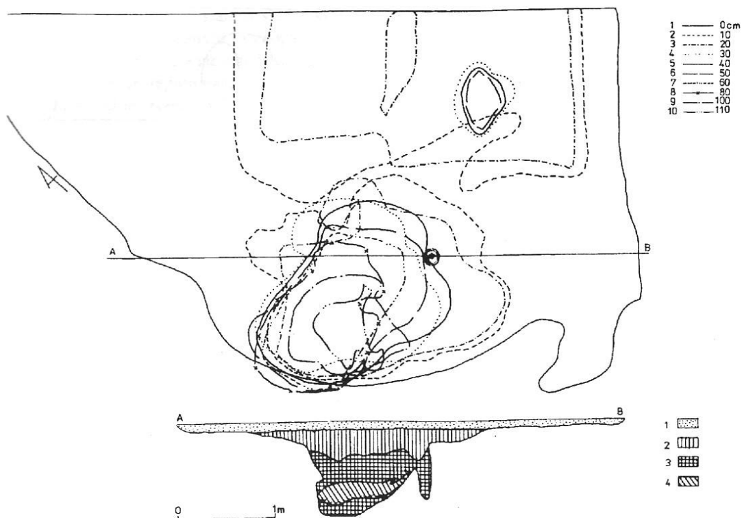
Рис. 9. Olchowa, gm. Iwierzycze, woj. podkarpackie, stanowisko 20. Rzut i profil obiektu 3; 1 – warstwa ciemnobieżowa, 2 – warstwa jasnobrunatna, 3 – warstwa ciemnobrunatna, 4 – warstwa czarnobrunatna
