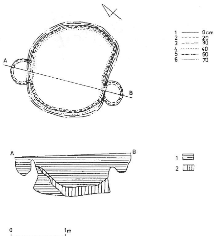
Рис. 9. Ольхова, гм. Ивежицы, воев. Подкарпатское, памятник 20. План и разрез объекта 3; 1 – темно-бежевый слой, 2 – светло-бурый слой, 3 – темно-бурый слой, 4 – черно-бурый слой
