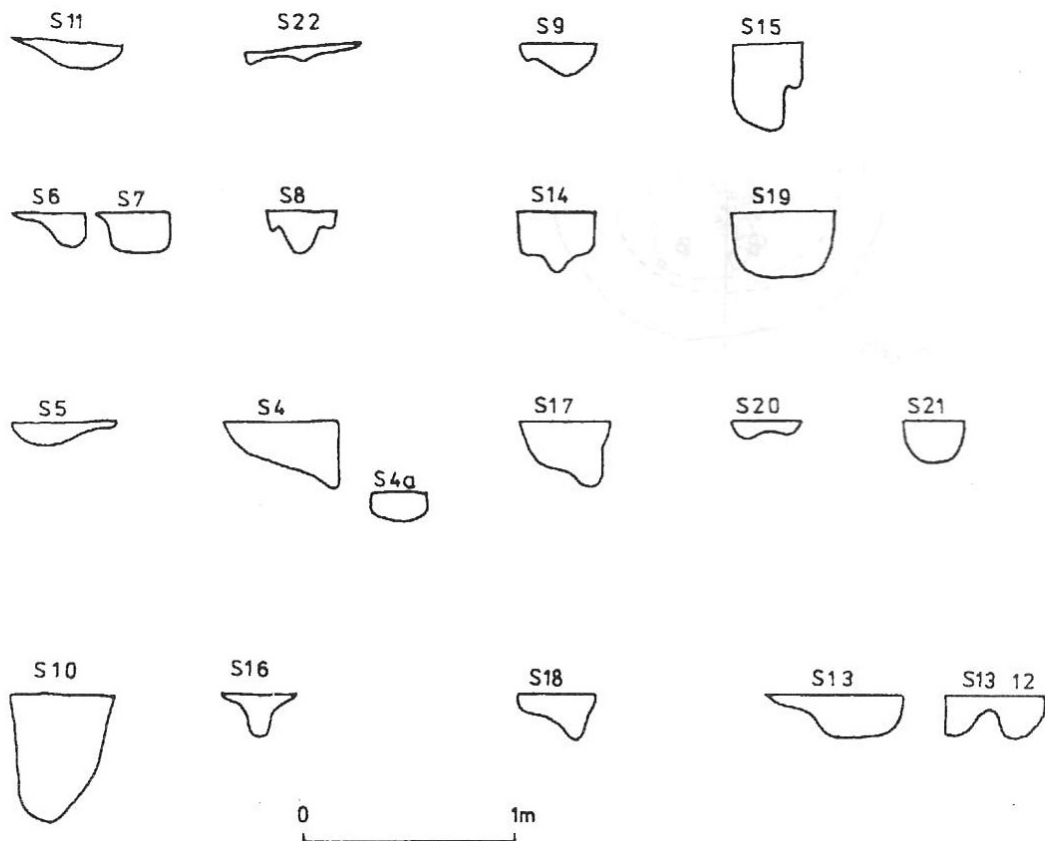
Рис. 12. Olchowa, gm. Iwierzycze, woj. podkarpackie, stanowisko 20. Profile dołków posłupowych z wykopu III
