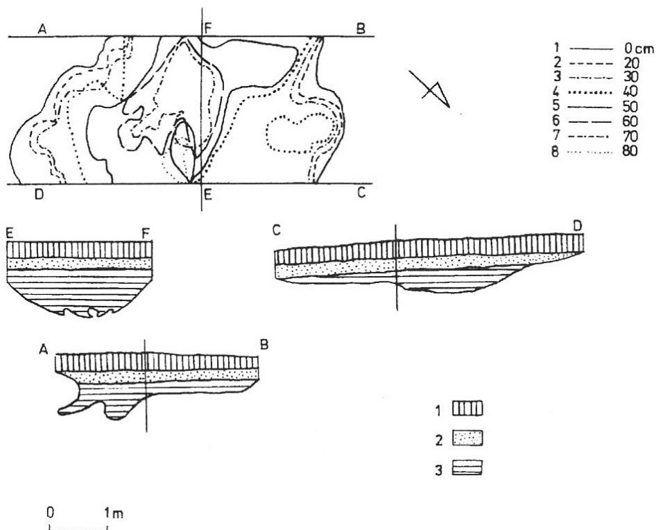
Рис. 11. Olchowa, gm. Iwierzycze, woj. podkarpackie, stanowisko 20. Rzut i profile obiektu 12; 1 – warstwa orna, 2 – warstwa brunatna, 3 – warstwa ciemnobrunatna
