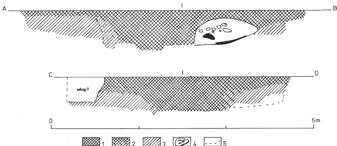
Ryc. 8. Grodzisko Dolne st. 8, woj. Rzeszów. Wykop IV, profile A-B i C-D obiektu 2. Oznaczenia: 1 – czarna ziemia; 2 – szarobrunatna ziemia; 3 – brązowożółta ziemia; 4 – destrukcja kamiennego pieca; 5 – słabo widoczna granica między żółtą ziemią o szarym nalocie i calcem
