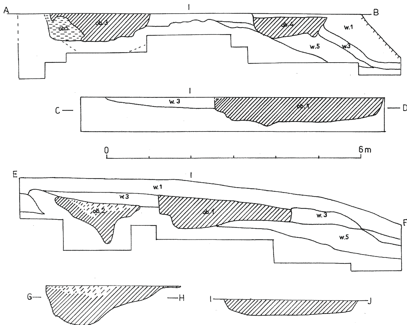
Ryc. 12. Grodzisko Dolne st. 28, woj. Rzeszów. Przekroje obiektów Abb. 12. Grodzisko Dolne Fundstelle 28, Wojewodschaft Rzeszów. Durchschnitte der Objekte Рис. 12. Гродзиско Дольне пам. 28, воев. Жешов. Разрезы объектов
