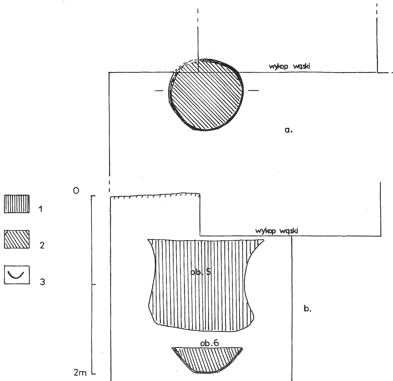
Ryc.13. Grodzisko Dolne st. 28, woj. Rzeszów. Rzut poziomy obiektu 6 (a) i profile obiektu 5 i 6 (b). Oznaczenia: 1 – szara ziemia ze żółtą; 2 – żółtopomarańczowa glina; 3 – polepa
