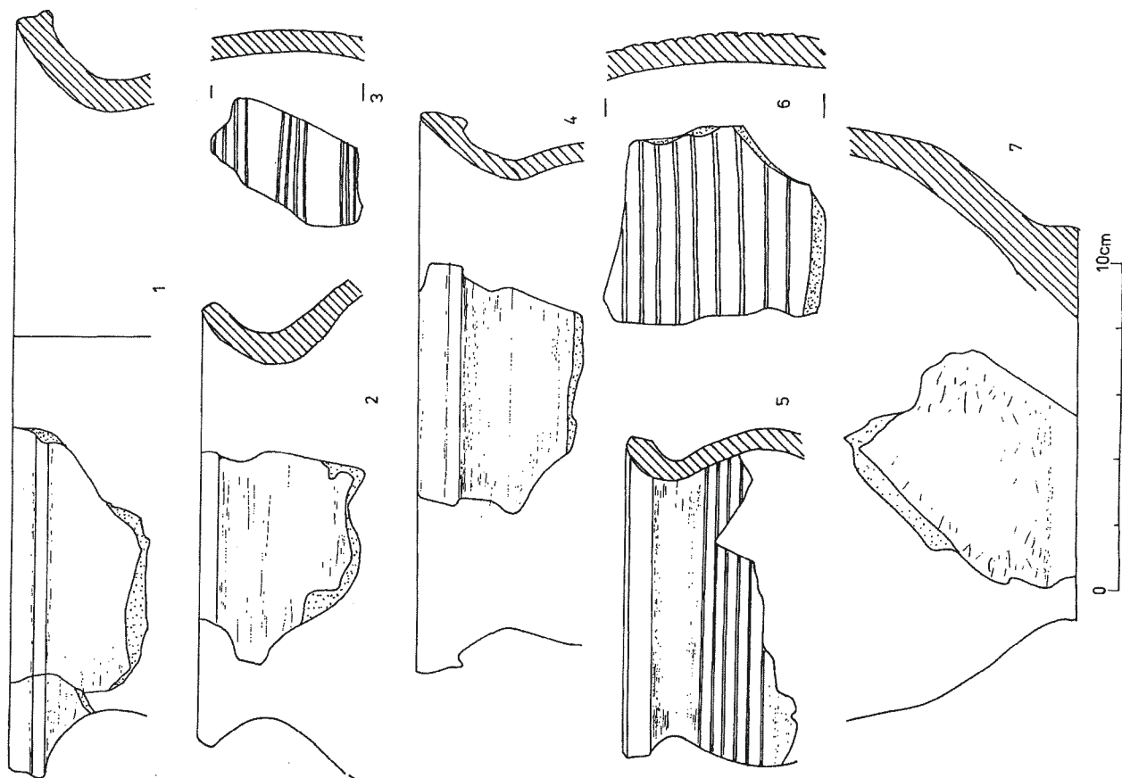
Tabl. II. Grodzisko Dolne st. 8, woj. Rzeszów. Wybór ceramiki z obiektu I Taf. II. Grodzisko Dolne Fundstelle 8, Wojewodschafft Rzeszów. Keramikauswahl aus dem Objekt I Табл. II. Гродзиско Дольне пам. 8, воєв. Жешов. Виборка кераміки из об'єкта I
