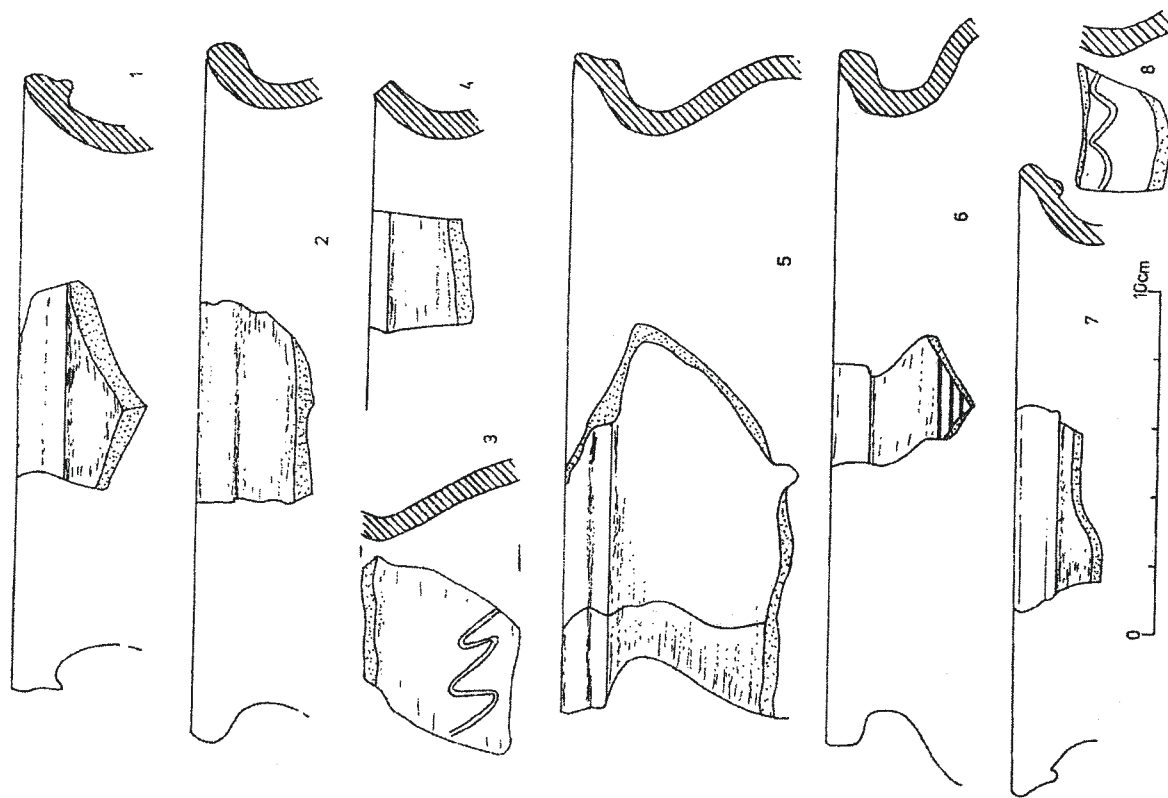
Tabl. IV. Grodzisko Dolne, woj. Rzeszów. Wybór ceramiki ze st. 8 – obiekt 5 (1–4) oraz ze st. 28 – warstwa kulturowa (5–8)
