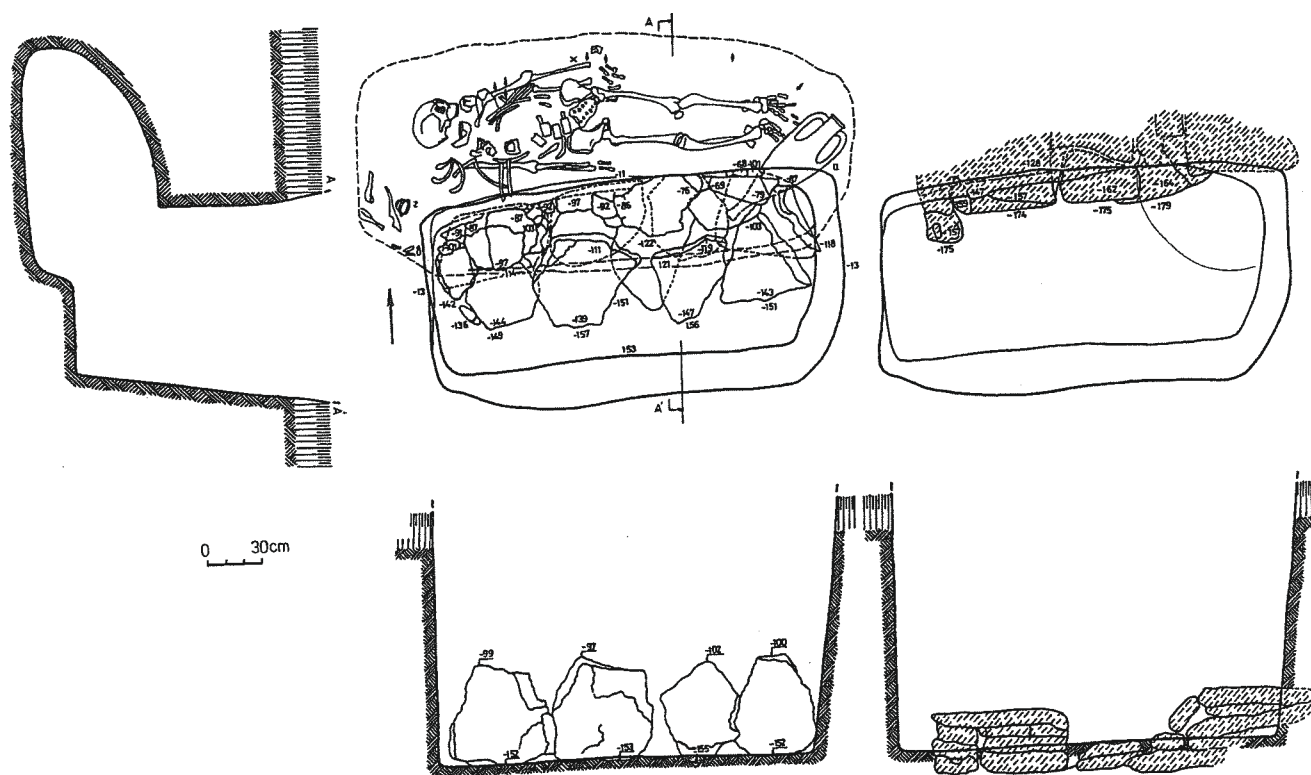
Ryc. 12. Grób 57 – plany i przekroje obiektu Abb. 12. Grab 57 – Pläne und Grundrisse des Objekts Рис. 12. Погребение 57 – планы и разрезы объекта
