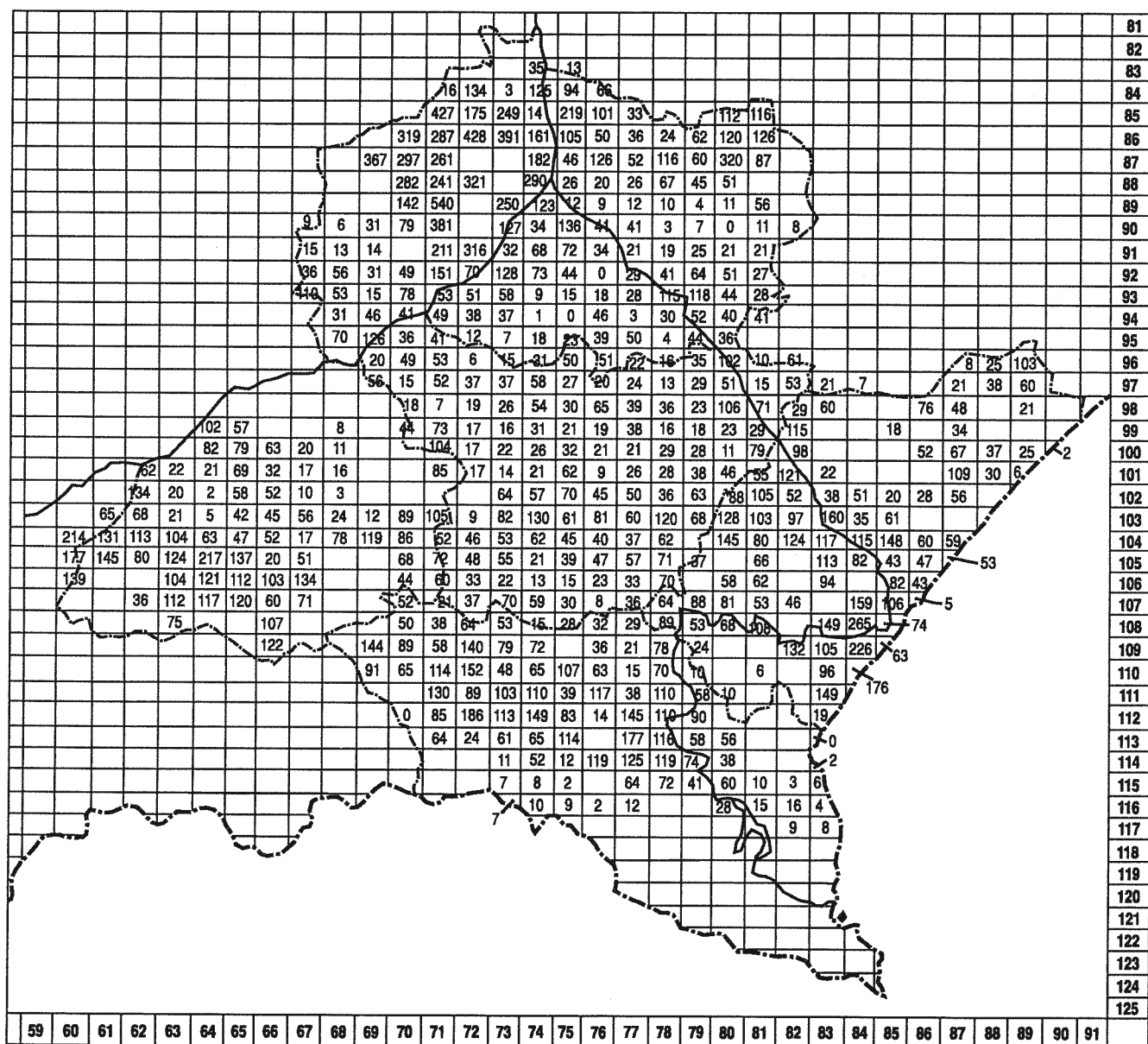
Ryc. 1. Stan zaawansowania Archeologicznego Zdjęcia Polski w pld.-wsch. Polsce (wg danych na koniec 1999 roku); obszary zbadane zaznaczono cyfrą pokazującą jednocześnie liczbę zewidencjonowanych stanowisk
