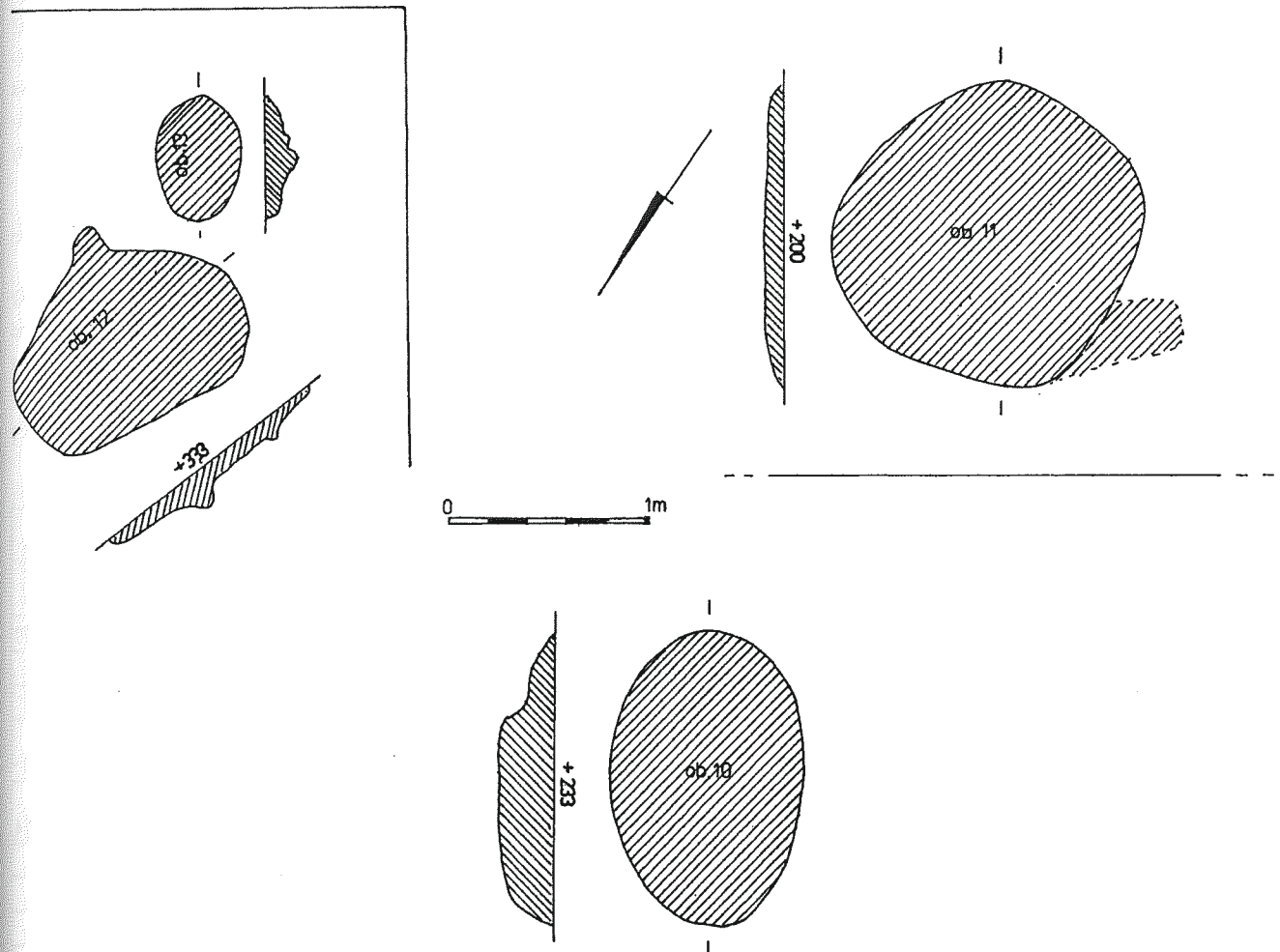
Ryc. 10. Wyżne, pow. Strzyżów, stan. 14. Rzuty i przekroje obiektów 10-13 Abb. 10. Wyżne, Kreis Strzyżów, Fundst. 14. Grundrisse und Profile der Objekte 10-13 Рис. 10. Выжное, пов. Стжижов, пам. 14. Планы и разрезы объектов 10-13
