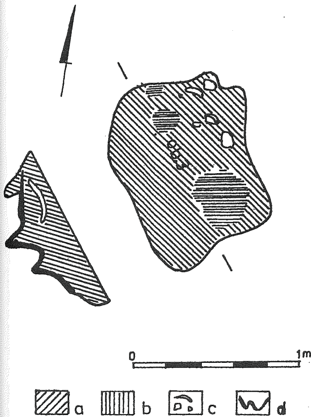
Ryc. 9. Wyżne, pow. Strzyżów, stan. 14. Ar 3W1S – rzut i przekrój obiektu 3. a – szaropopielata glina; b – ciemnoszara ziemia; c – większe fragmenty ceramiki; d – warstwa spalenizny przy dnie obiektu
