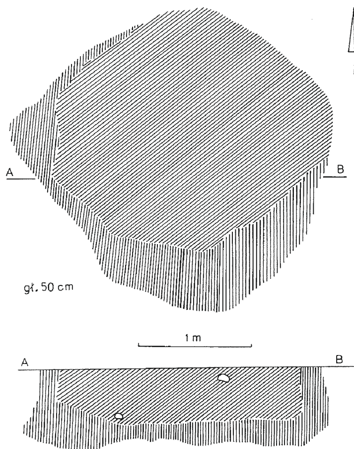
Ryc. 12. Radymno, pow. Jarosław, st. 12. Rzut poziomy i profil obiektu 13 Abb. 12. Radymno, Kreis Jarosław, Fundst. 12. Grundriß und Profil des Objekts 13 Рис. 12. Радымно, пов. Ярослав, пам. 12. План и разрез объекта 13
