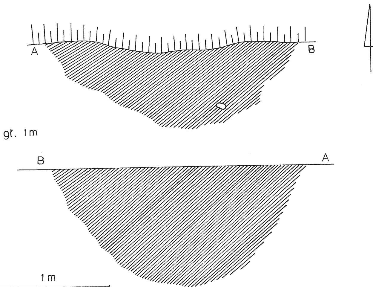
Ryc. 7. Radymno, pow. Jarosław, st. 12. Rzut poziomy i profil obiektu 6
