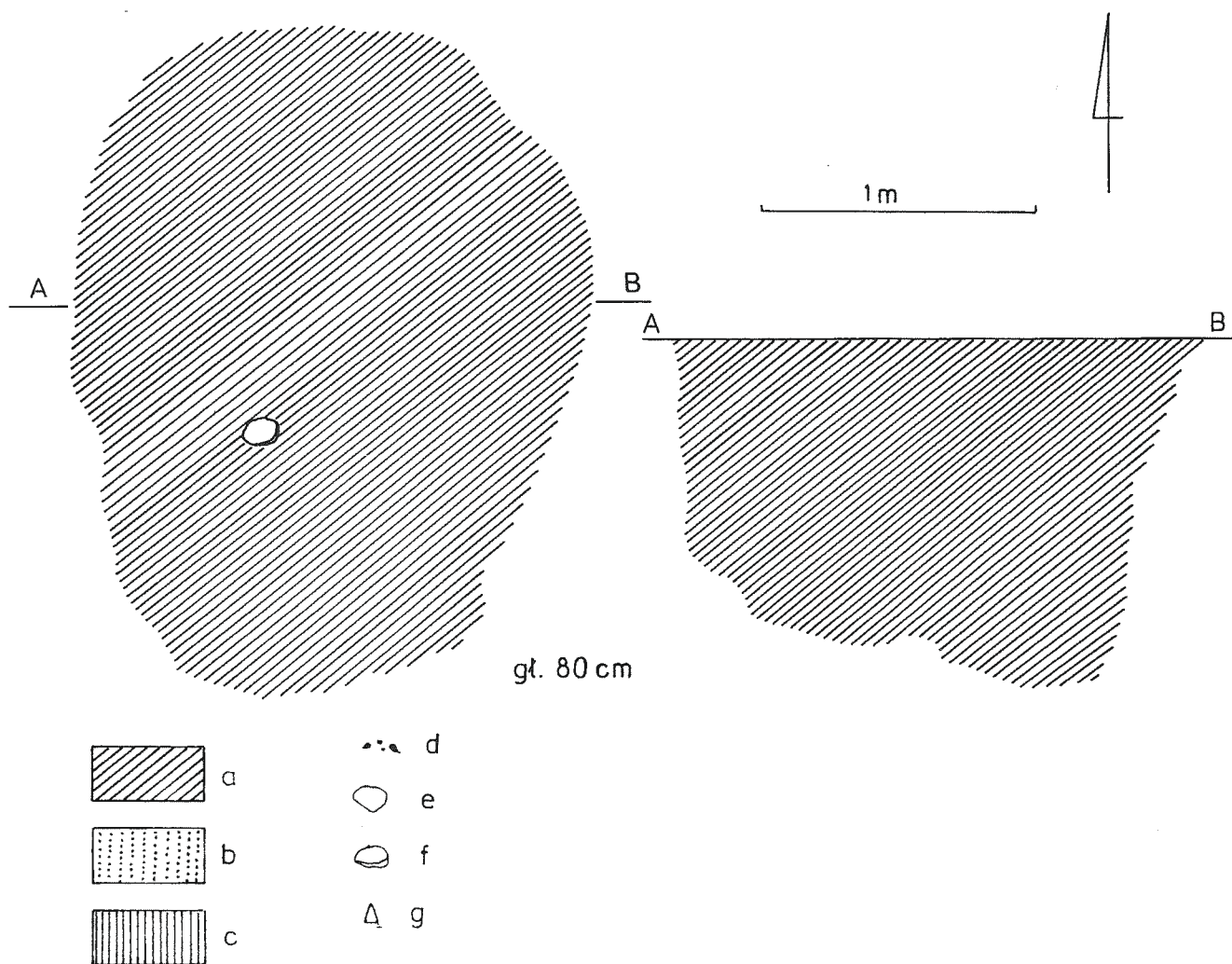
Ryc. 3. Radymno, pow. Jarosław, st. 12. Rzut poziomy i profil obiektu 1: a – ziemia czarna, b – warstwa z popiołem, c – ziemia brunatna, d – węgiel drzewny, e – polepa, f – kamienie, g – ceramika
