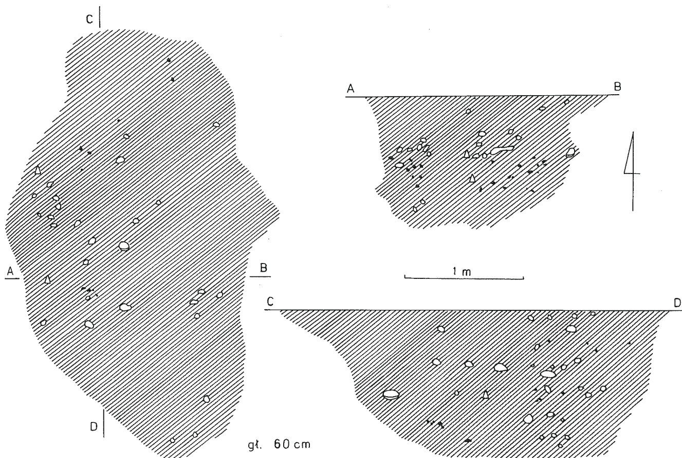
Ryc. 8. Radymno, pow. Jarosław, st. 12. Rzut poziomy i profile obiektu 9
