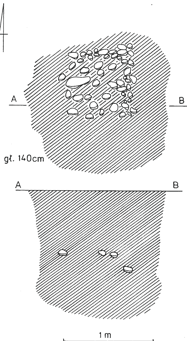
Ryc. 5. Radymno, pow. Jarosław, st. 12. Rzut poziomy i profil obiektu 3
