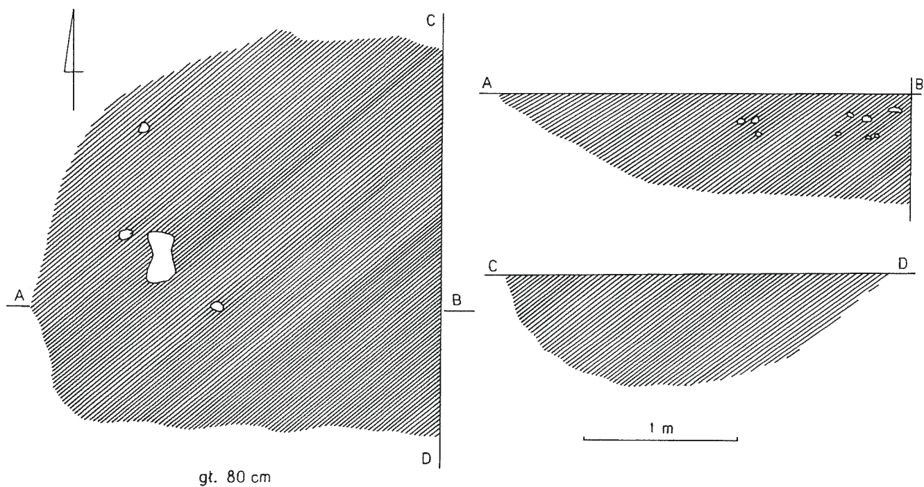
Ryc. 10. Radymno, pow. Jarosław, st. 12. Rzut poziomy i profile obiektu 11
