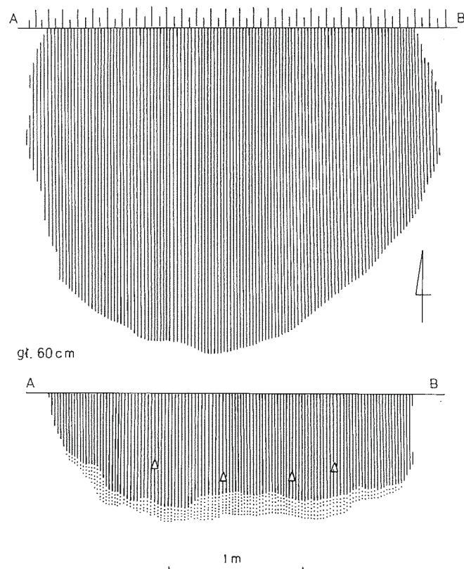
Ryc. 5. Radymno, pow. Jarosław, st. 12. Rzut poziomy i profil obiektu 3
