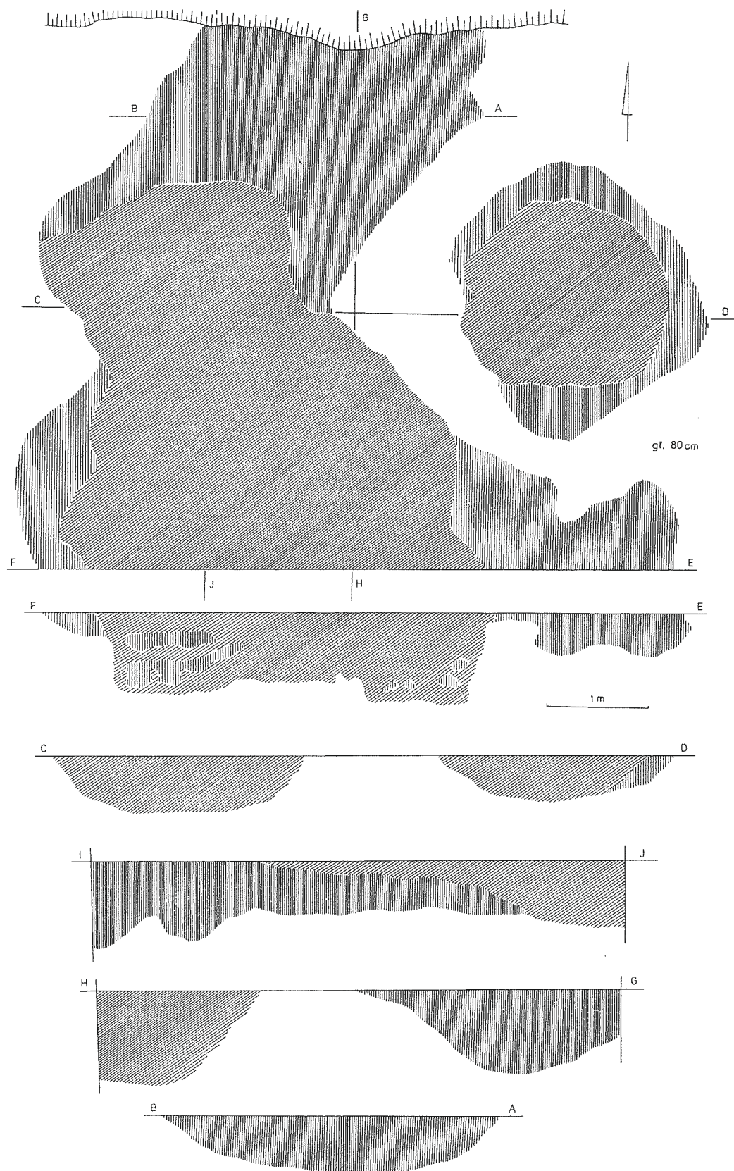
Ryc. 11. Radymno, pow. Jarosław, st. 12. Rzut poziomy i profile obiektu 12 oraz 14 i 15 Abb. 11. Radymno, Kreis Jaroslaw, Fundst. 12. Grundriß und Profile der Objekte 12, 14 und 15 Рис. 11. Радымно, пов. Ярослав, пам. 12. План и разрезы объектов 12, 14, 15
