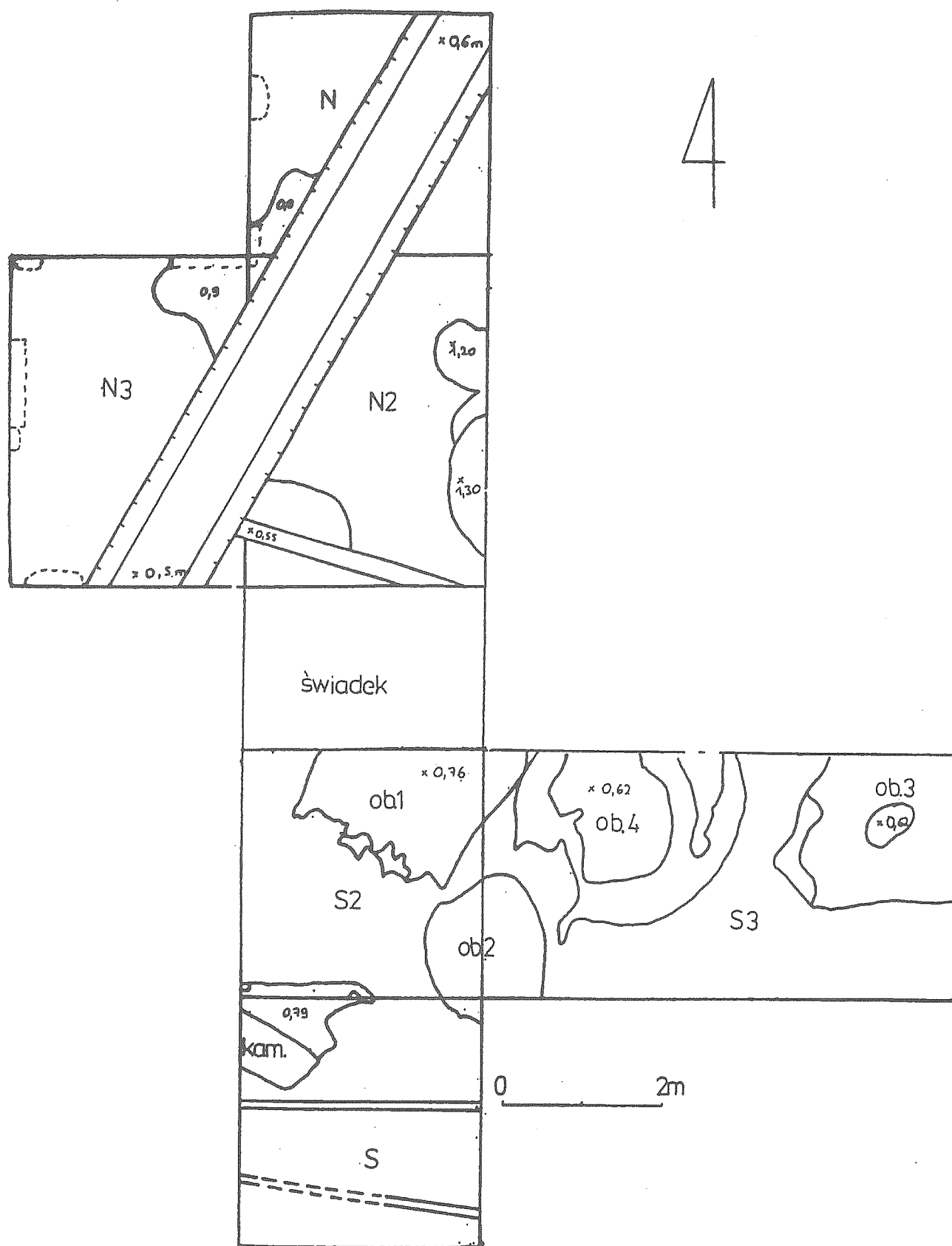
Ryc. 1. Rzeszów, ul. Słowackiego. Rozplanowanie wykopów z naniesionymi obiektami i kanałem kanalizacyjnym Abb. 1. Rzeszów, Słowacki – Straße. Verteilung der Grabungsschnitte mit den markierten Objekten und dem Kanalisationskanal Рис. 1. Жешов, ул. Словацкого. Планировка раскопов с нанесенными объектами и канализационным туннелем
