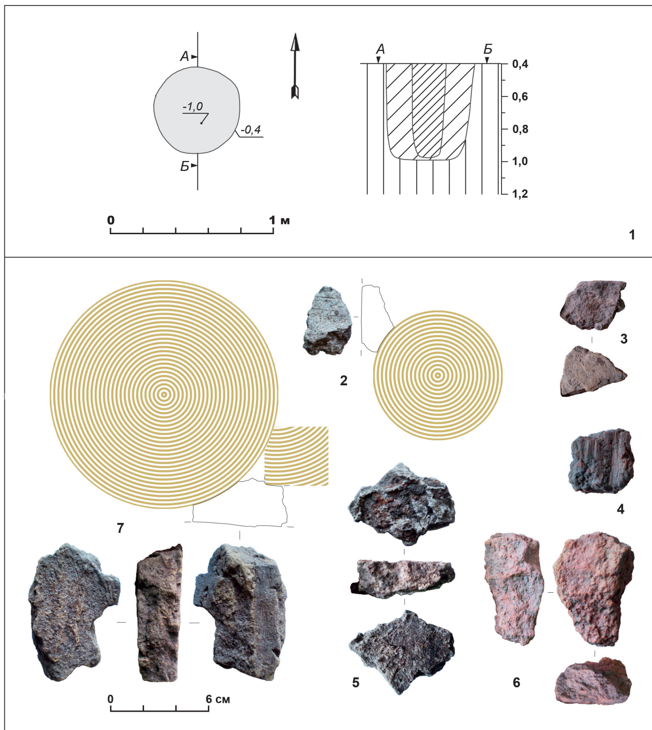
Рис. 31. Шацьк – ур. Сад. 2011. Розкоп 4. 1 – план і розріз об'єкту 57; 2–7 – вибірка фрагментів обмазки з об'єкту 57 Abb. 31. Szack – Fst. Sad. 2011. Grabungsschnitt 4. 1 – Plan und Profil des Objekts 57; 2–7 – Fragmente des Hüttenlehms aus dem Objekt 57 – Auswahl
