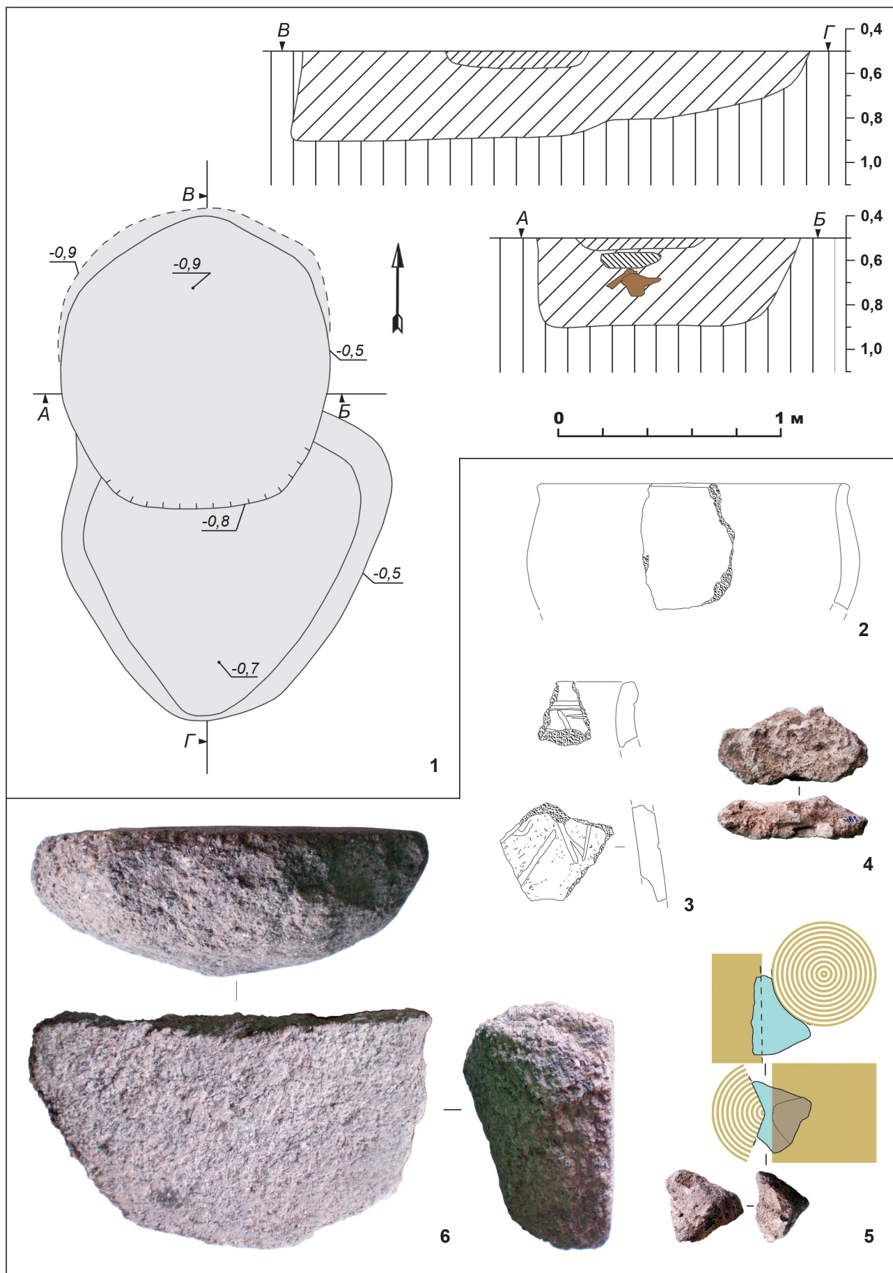
Рис. 32. Шацьк – ур. Сад. 2011. Розкоп 4. 1 – план і розрізи об'єкту 59; 2–6 – вибірка матеріалів з об'єкту 59
