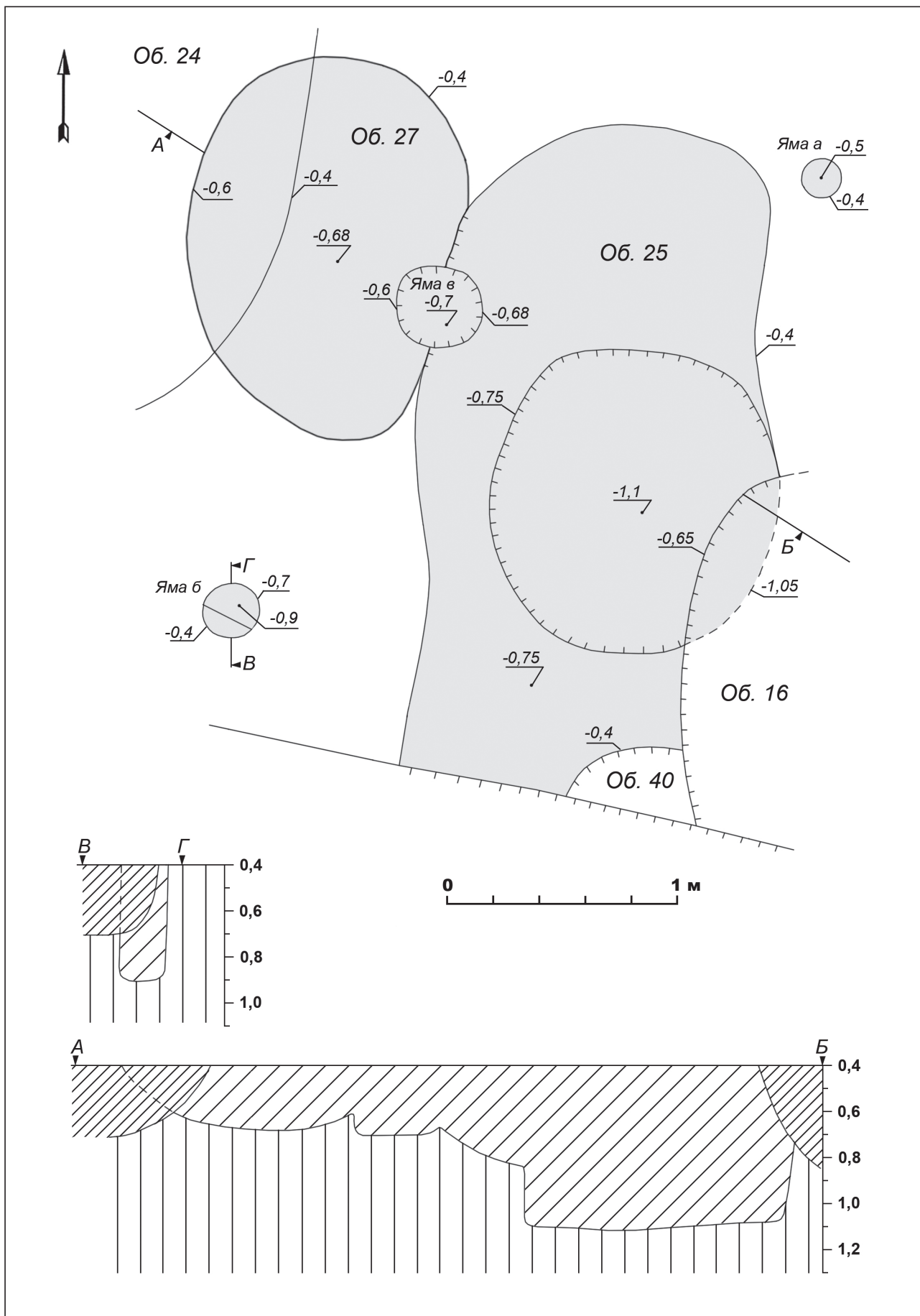
Рис. 21. Шацьк – ур. Сад. 2011. Розкоп 4. План і розрізи об'єктів 25 і 27
