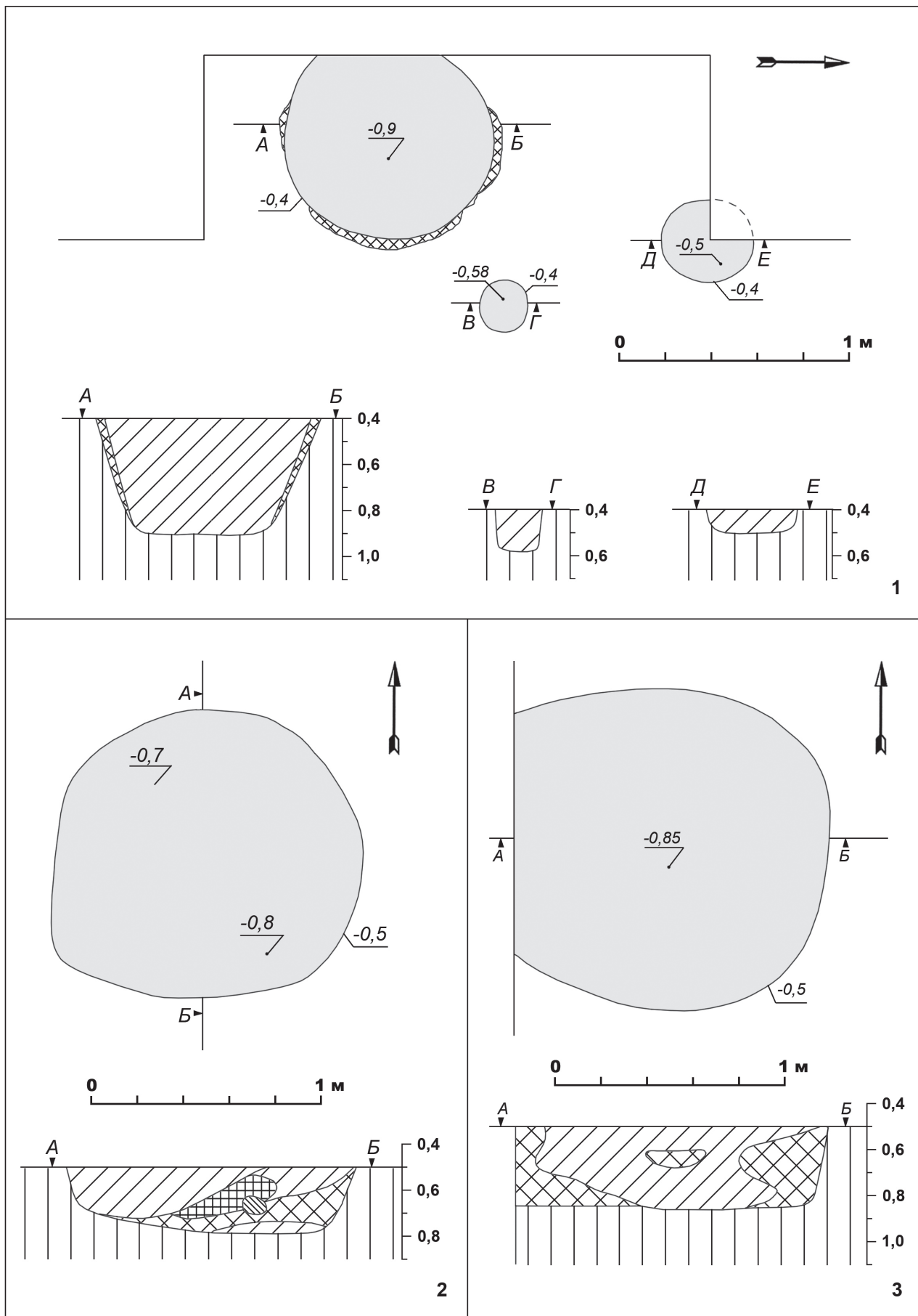
Рис. 26. Шацьк – ур. Сад. 2011. Розкоп 4. 1 – план і розрізи об'єкту 44; 2 – план і розріз об'єкту 58; 3 – план і розріз об'єкту 68 Abb. 26. Szack – Fst. Sad. 2011. Grabungsschnitt 4. 1 – Plan und Profile des Objekts 44; 2 – Plan und Profil des Objekts 58; 3 – Plan und Profil des Objekts 68
