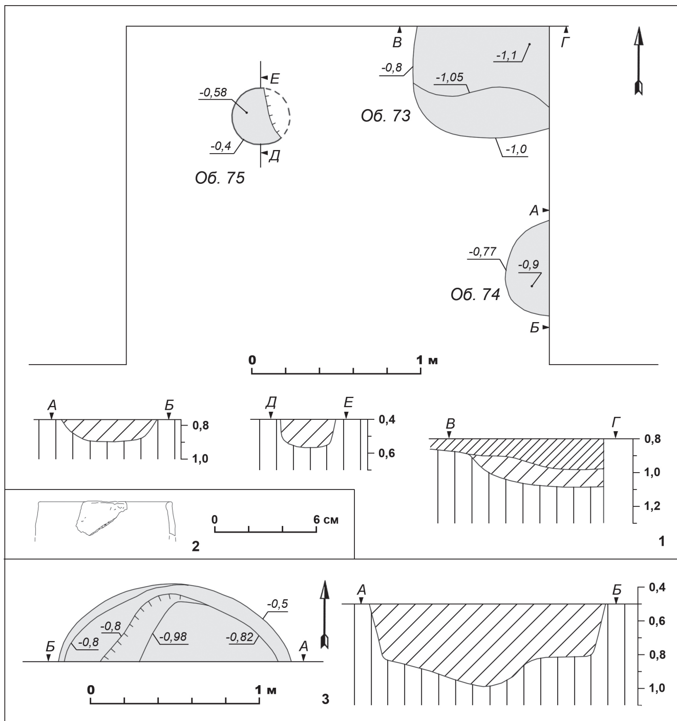
Рис. 38. Шацьк – ур. Сад. 2011. Розкоп 4. 1 – план і розрізи об'єктів 73, 74 і 75; 2 – фрагмент кераміки з об'єкту 74; 3 – план і розріз об'єкту 72
