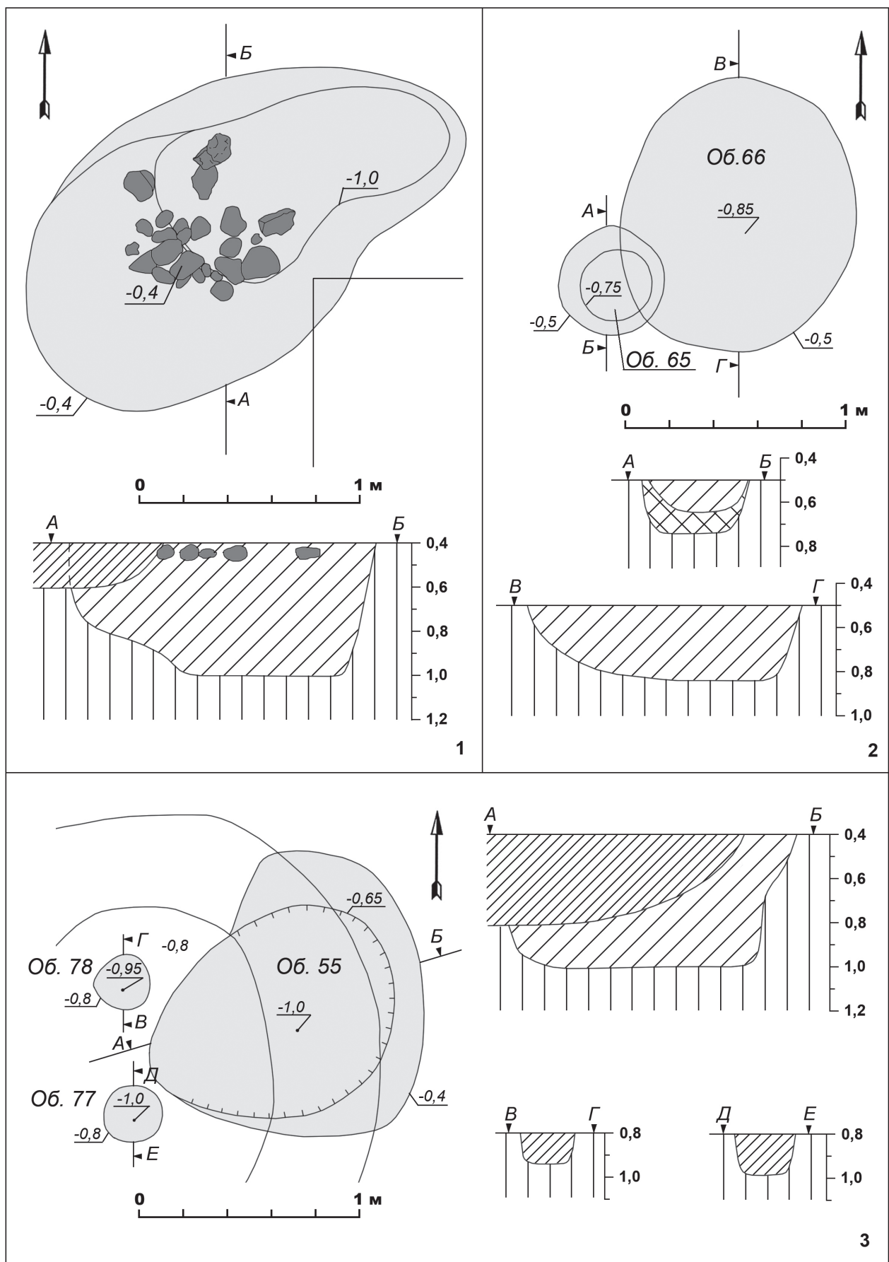
Рис. 29. Шацьк – ур. Сад. 2011. Розкоп 4. 1 – план і розріз об'єкту 53; 2 – план і розрізи об'єктів 65 і 66; 3 – план і розрізи об'єктів 55, 78 і 79
