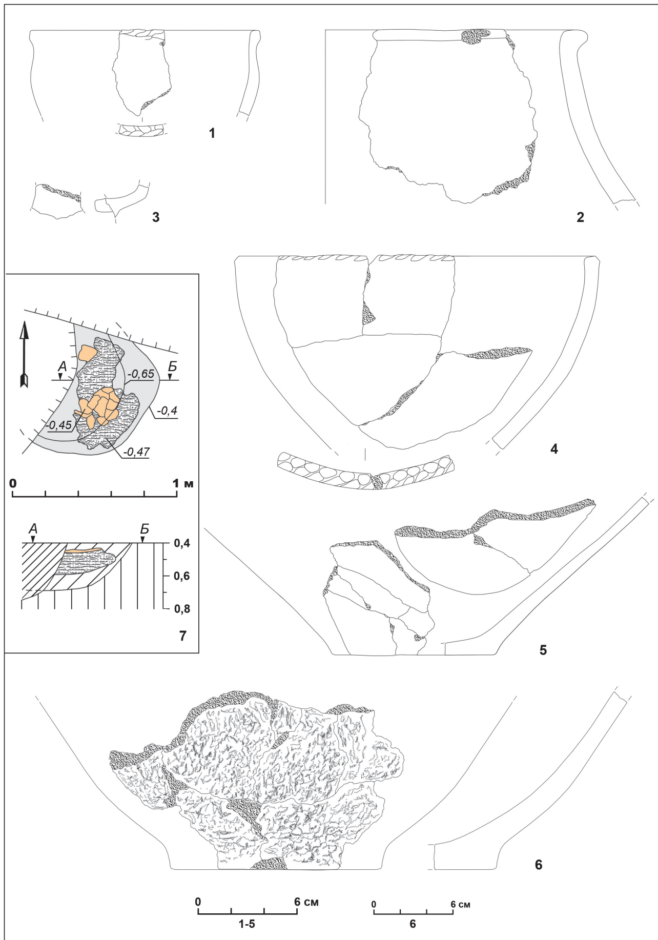
Рис. 19. Шацьк – ур. Сад. 2011. Розкоп 4. 1–6 – вибірка кераміки з об'єкту 21; 7 – план і розріз об'єкту 21 Abb. 19. Szack – Fst. Sad. 2011. Grabungsschnitt 4. 1–6 – Keramikauswahl aus dem Objekt 21; 7 – Plan und Profil des Objekts 21
