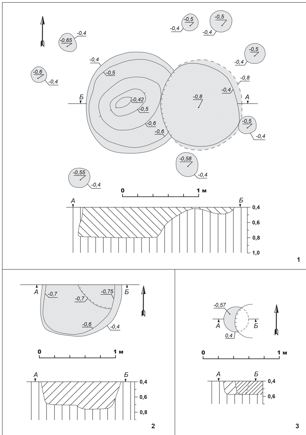
Рис. 25. Шацьк – ур. Сад. 2011. Розкоп 4. 1 – план і розріз об'єкту 34; 2 – план і розріз об'єкту 30; 3 – план і розріз об'єкту 49 Abb. 25. Szack – Fst. Sad. 2011. Grabungsschnitt 4. 1 – Plan und Profil des Objekts 34; 2 – Plan und Profil des Objekts 30; 3 – Plan und Profil des Objekts 49
