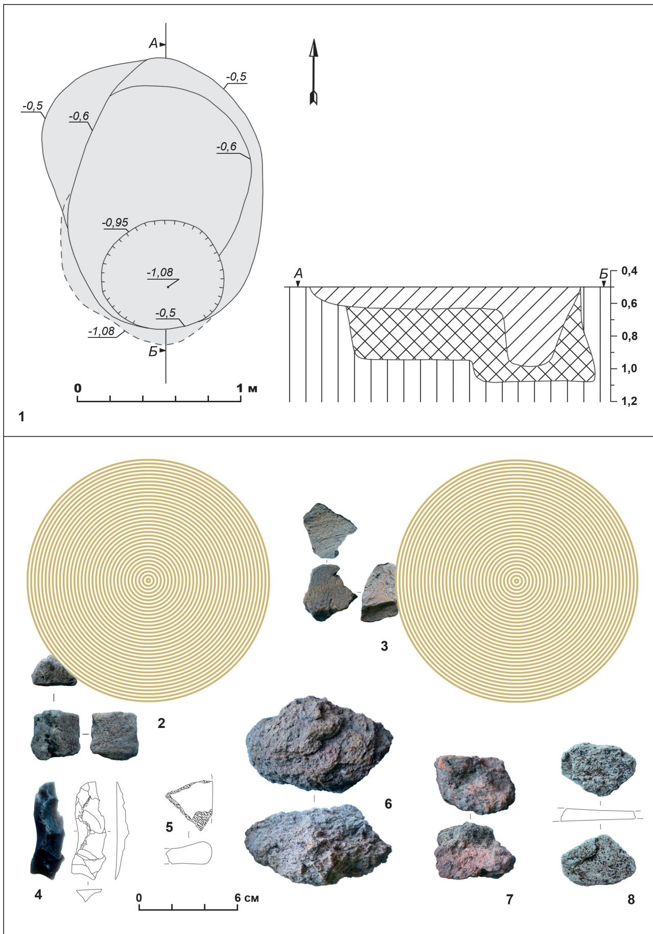
Рис. 33. Шацьк – ур. Сад. 2011. Розкоп 4. 1 – план і розріз об'єкту 60; 2–8 – вибірка матеріалів з об'єкту 60 Abb. 33. Szack – Fst. Sad. 2011. Grabungsschnitt 4. 1 – Plan und Profil des Objekts 60; 2–8 – Funde aus dem Objekt 60 – Auswahl
