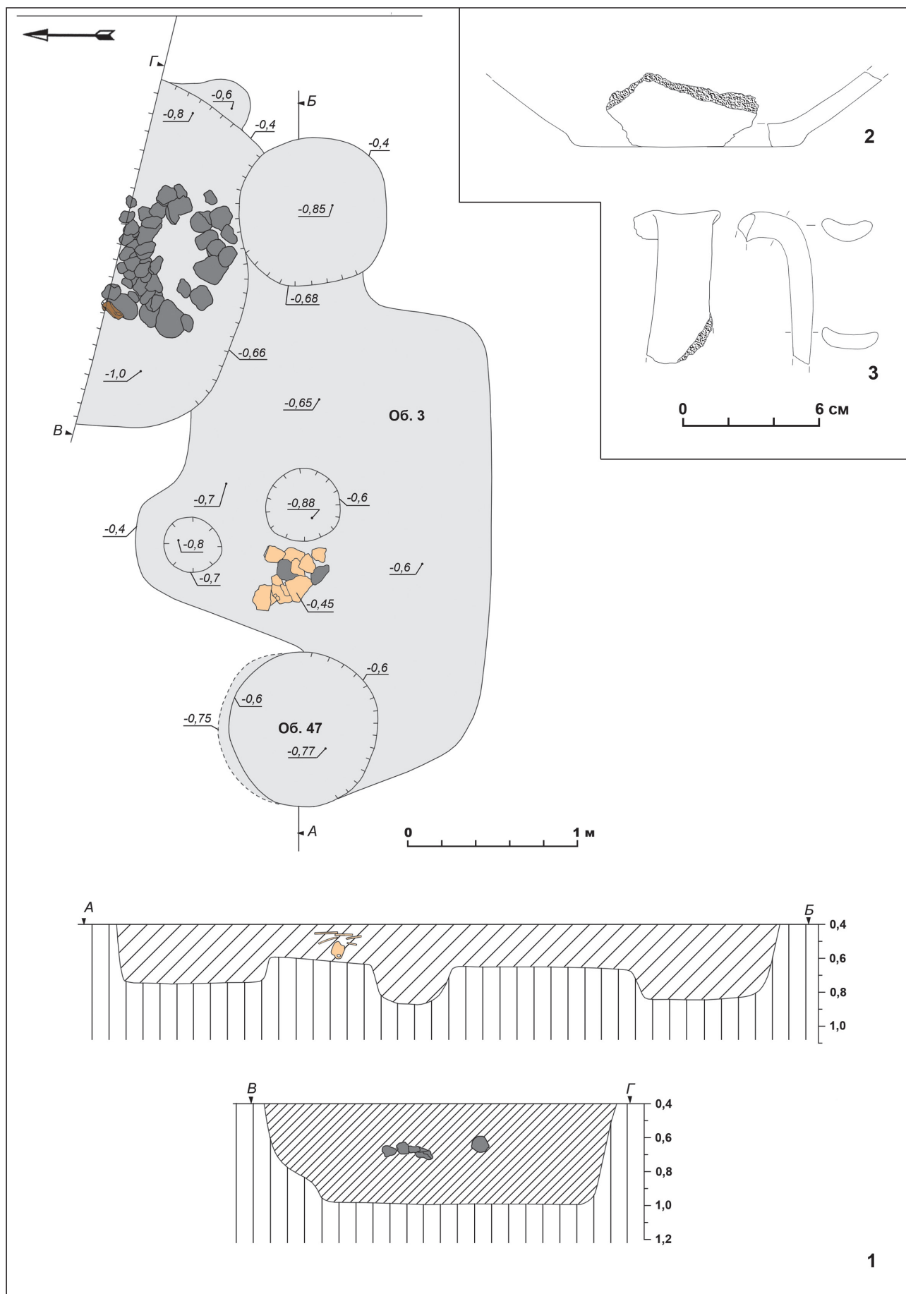
Рис. 7. Шацьк – ур. Сад. 2011. Розкоп 4. 1 – план і розрізи об'єктів 3 і 47; 2 – кераміка з об'єкту 47
