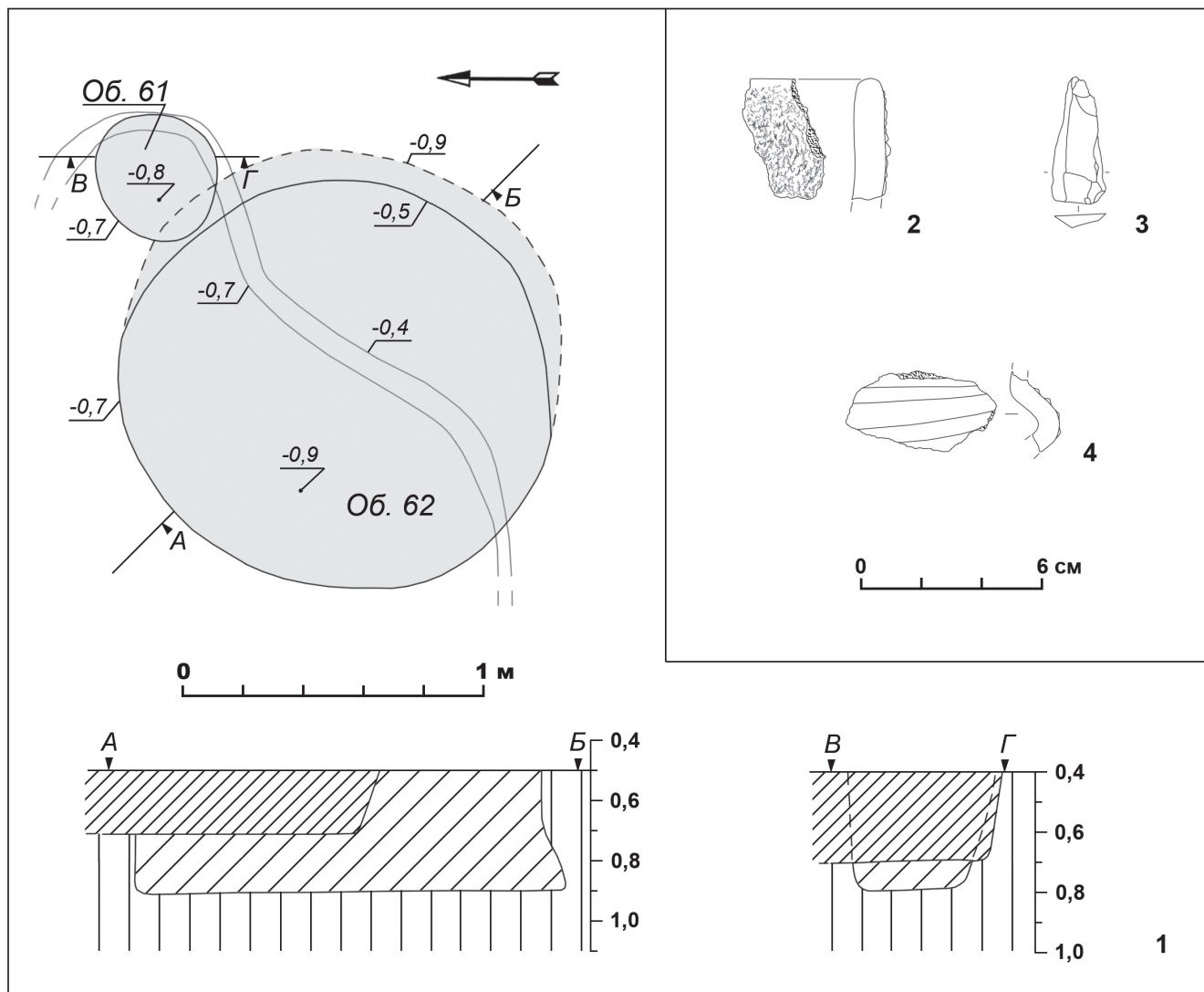
Рис. 34. Шацьк – ур. Сад. 2011. Розкоп 4. 1 – план і розрізи об'єктів 61 і 62; 2–4 – вибірка матеріалів з об'єкту 62 Abb. 34. Szack – Fst. Sad. 2011. Grabungsschnitt 4. 1 – Plan und Profile der Objekte 61 und 62; 2–4 – Funde aus dem Objekt 62 – Auswahl
