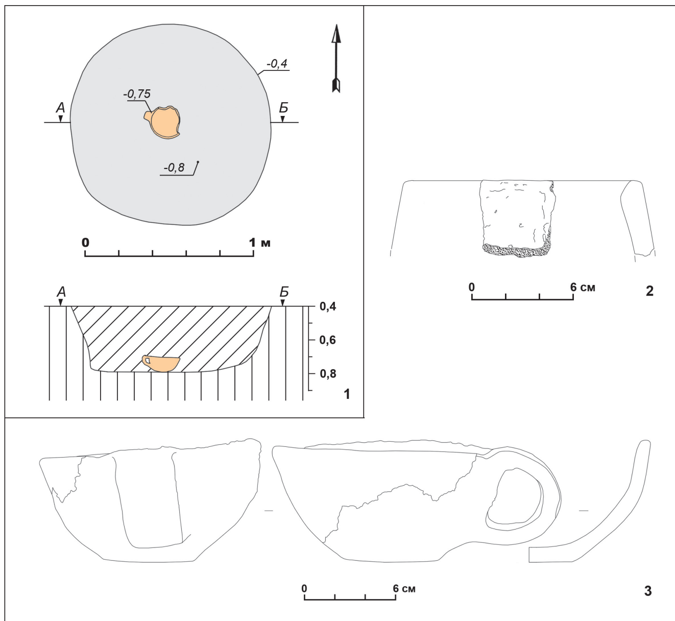
Рис. 12. Шацьк – ур. Сад. 2011. Розкоп 4. 1 – План і розріз об'єкту 9; 2, 3 – кераміка з об'єкту 9
