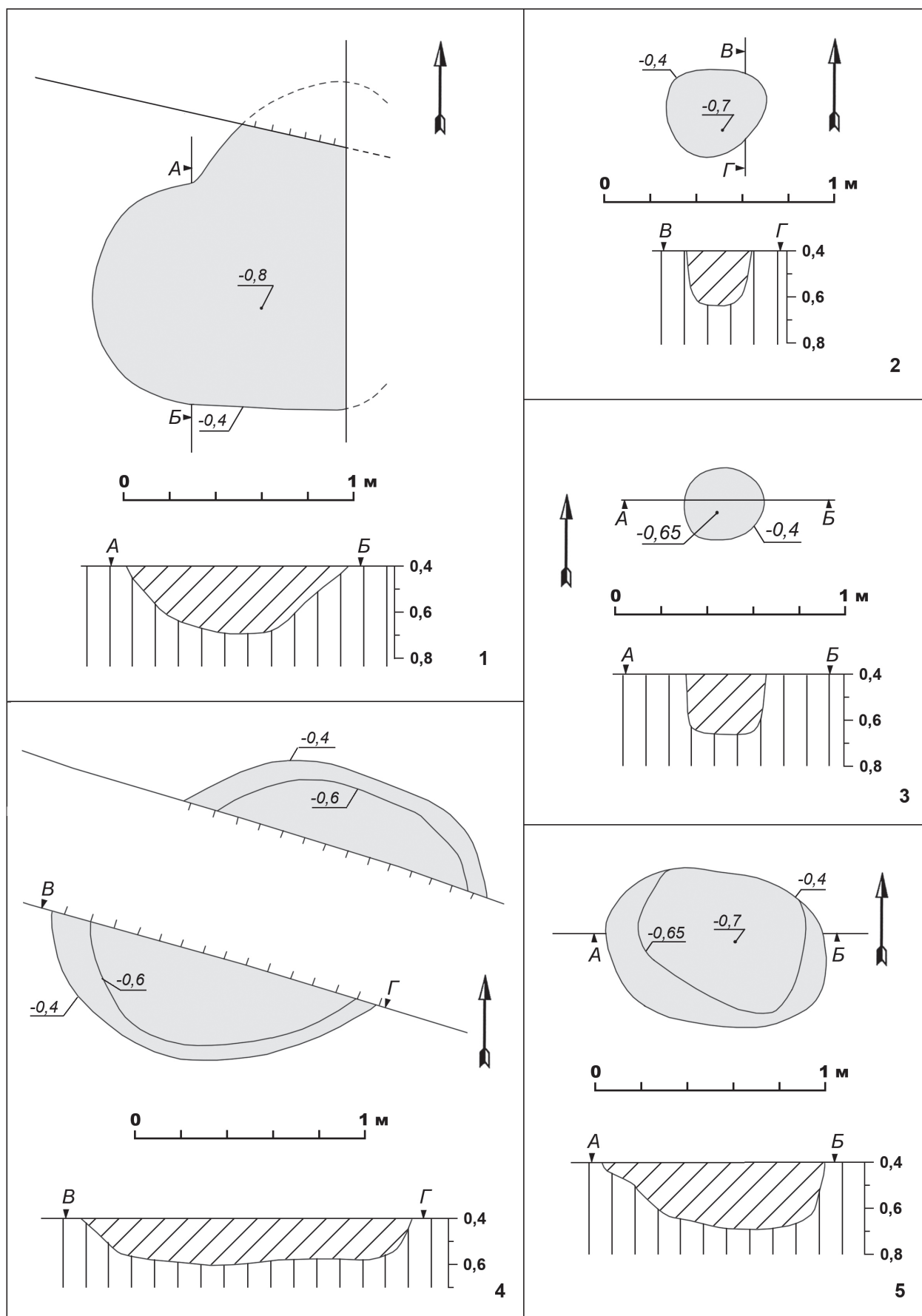
Рис. 14. Шацьк – ур. Сад. 2011. Розкоп 4. 1 – план і розріз об'єкту 11; 2 – план і розріз об'єкту 12; 3 – план і розріз об'єкту 23; 4 – план і розріз об'єкту 28; 5 – план і розріз об'єкту 36
